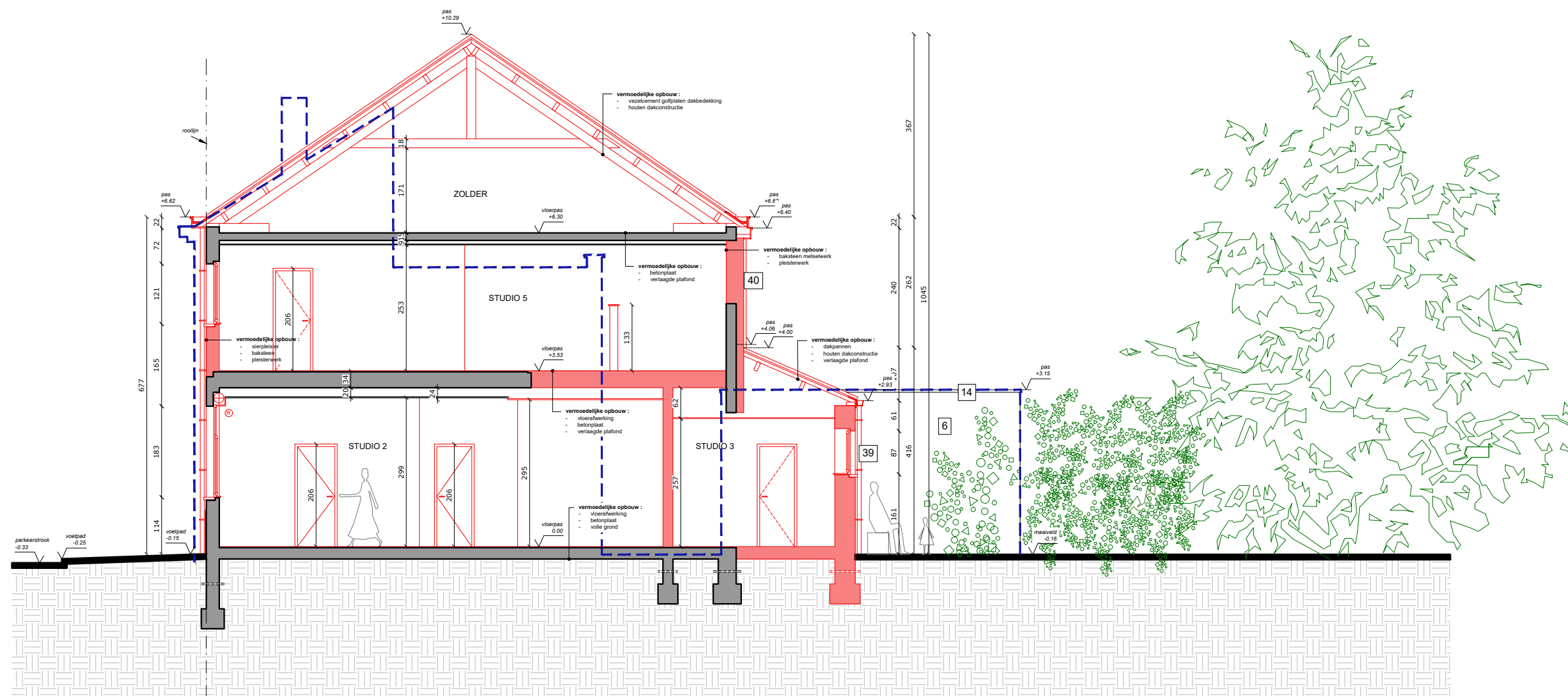
DOORSNEDE BB
