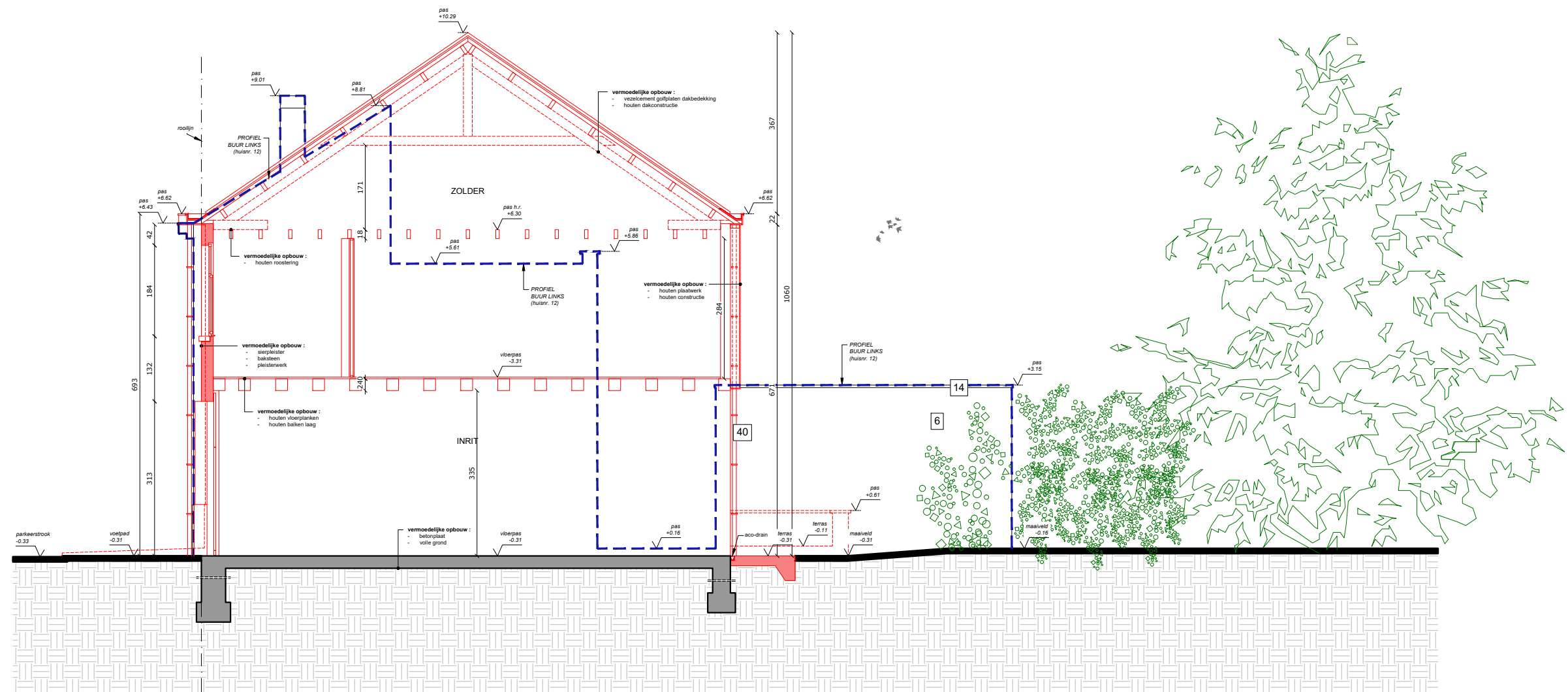
DOORSNEDE CC
