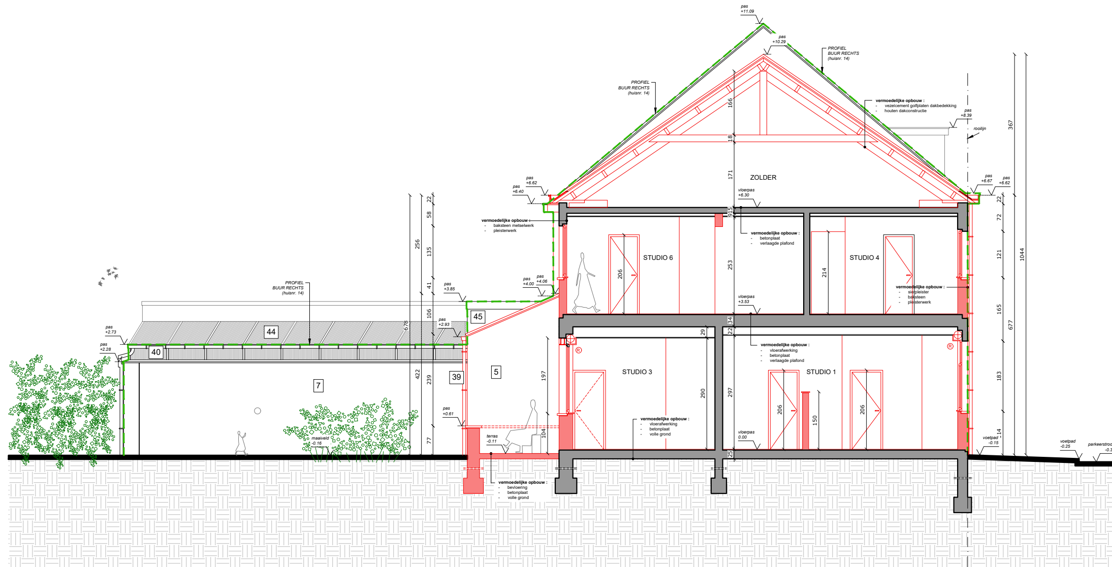
DOORSNEDE AA
