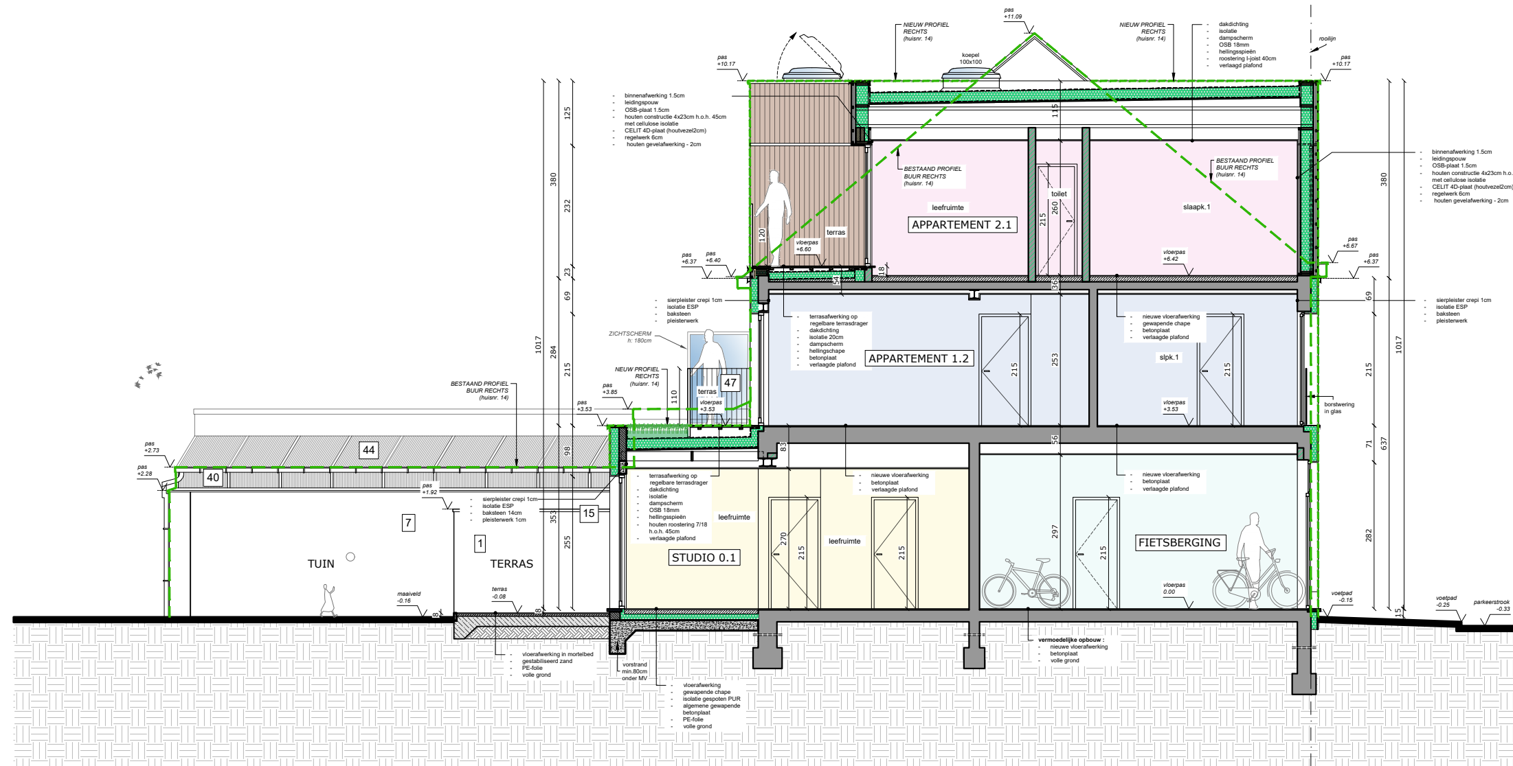
DOORSNEDE AA
