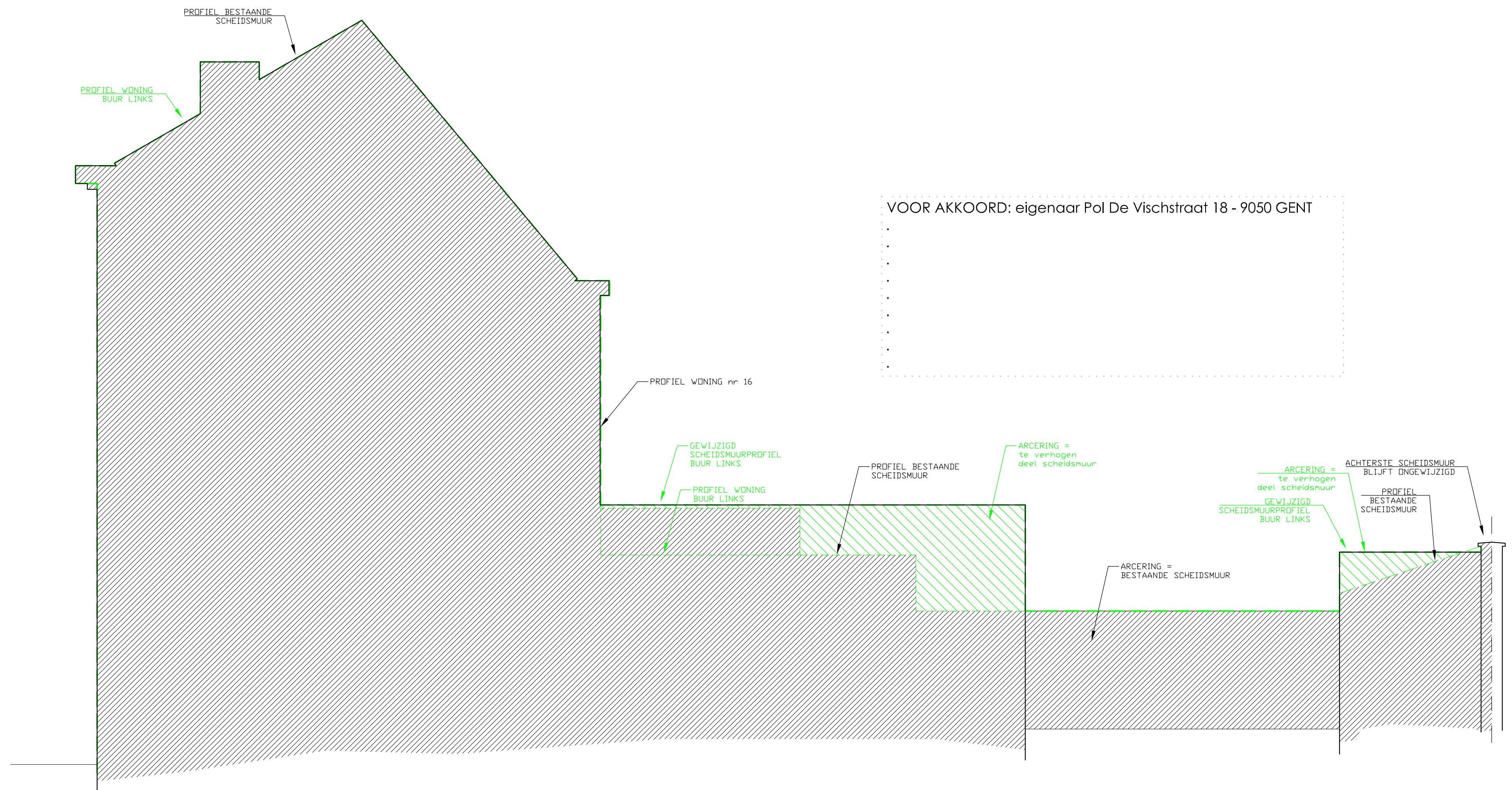
SCHEIDSMUURPROFIEL LINKS
