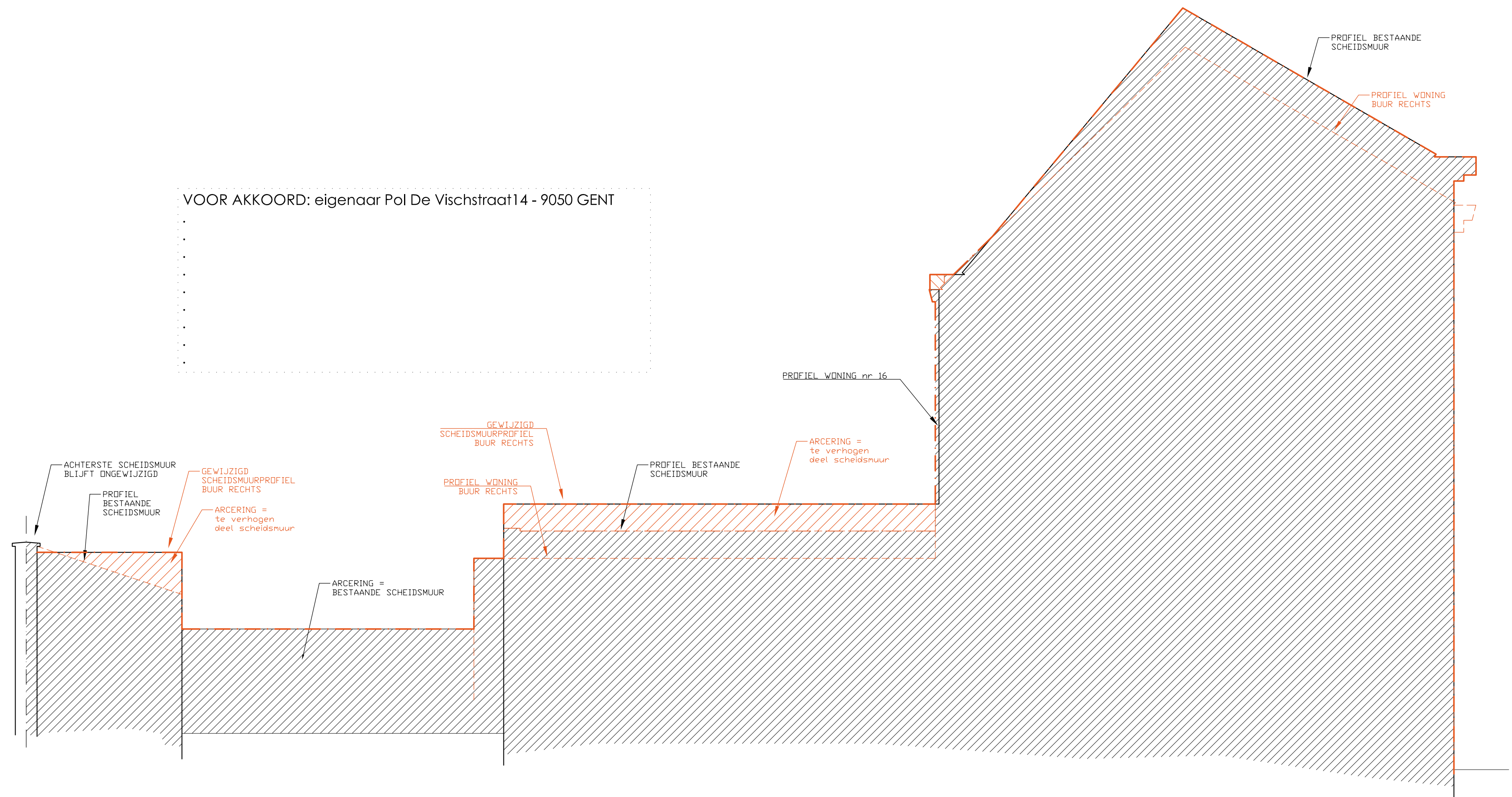
SCHEIDSMUURPROFIEL RECHTS
