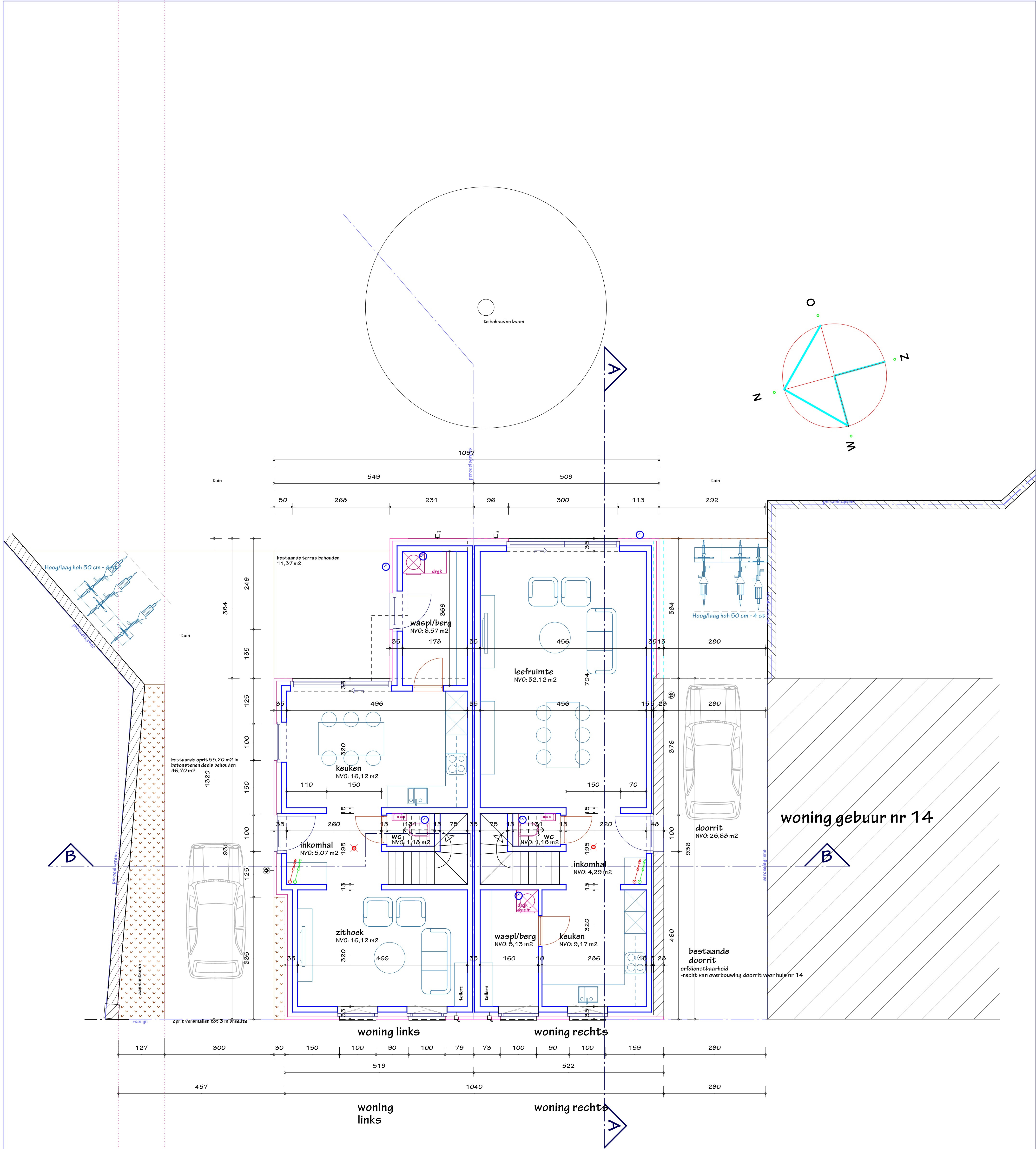
GRONDPLAN
