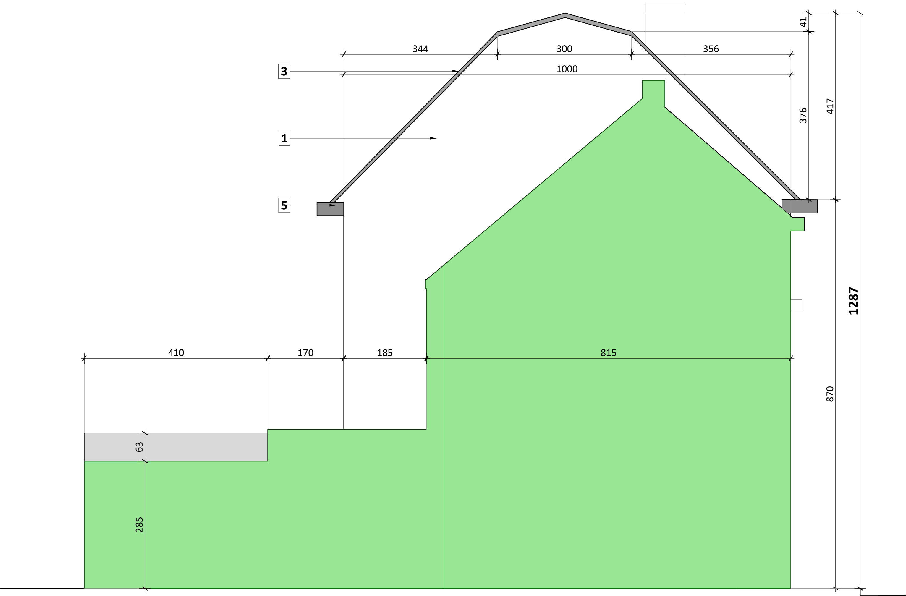
zijgevel links nieuwe toestand = bestaande toestand na regularisatie
