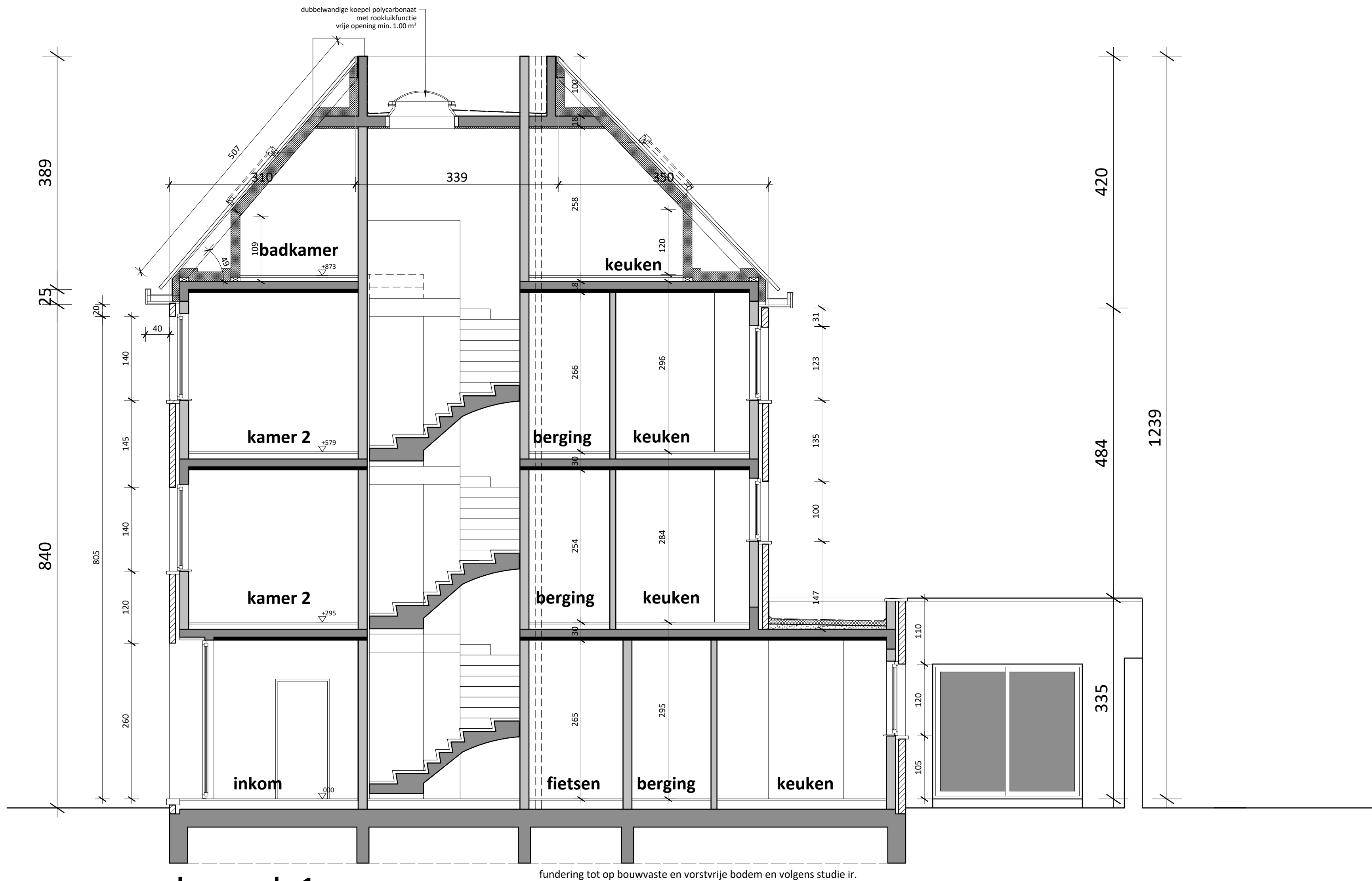
doorsnede 1 vergunde toestand
