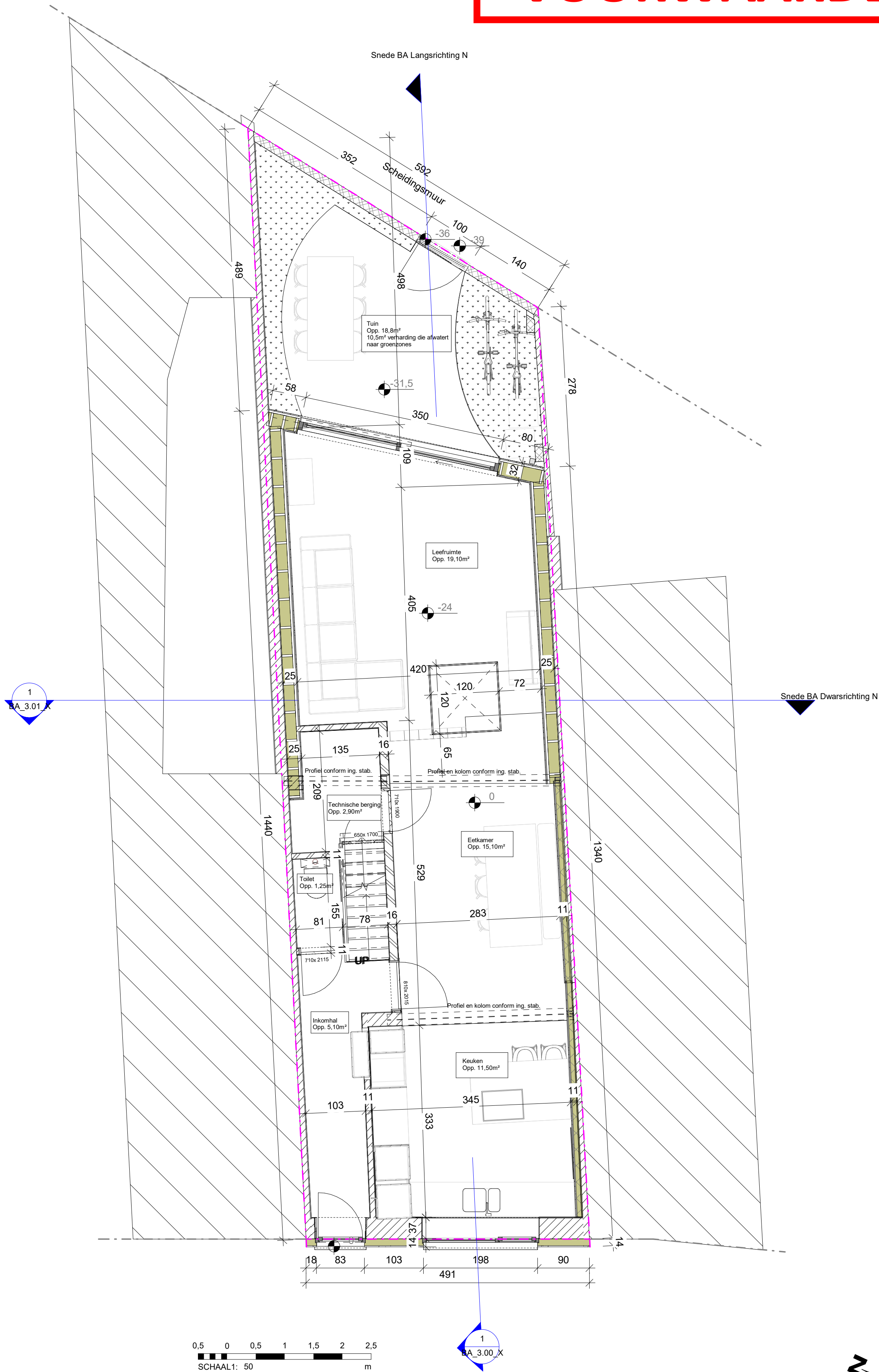
BA_1.00_X P_N_1.00_Grondplan Gelijkvloers
