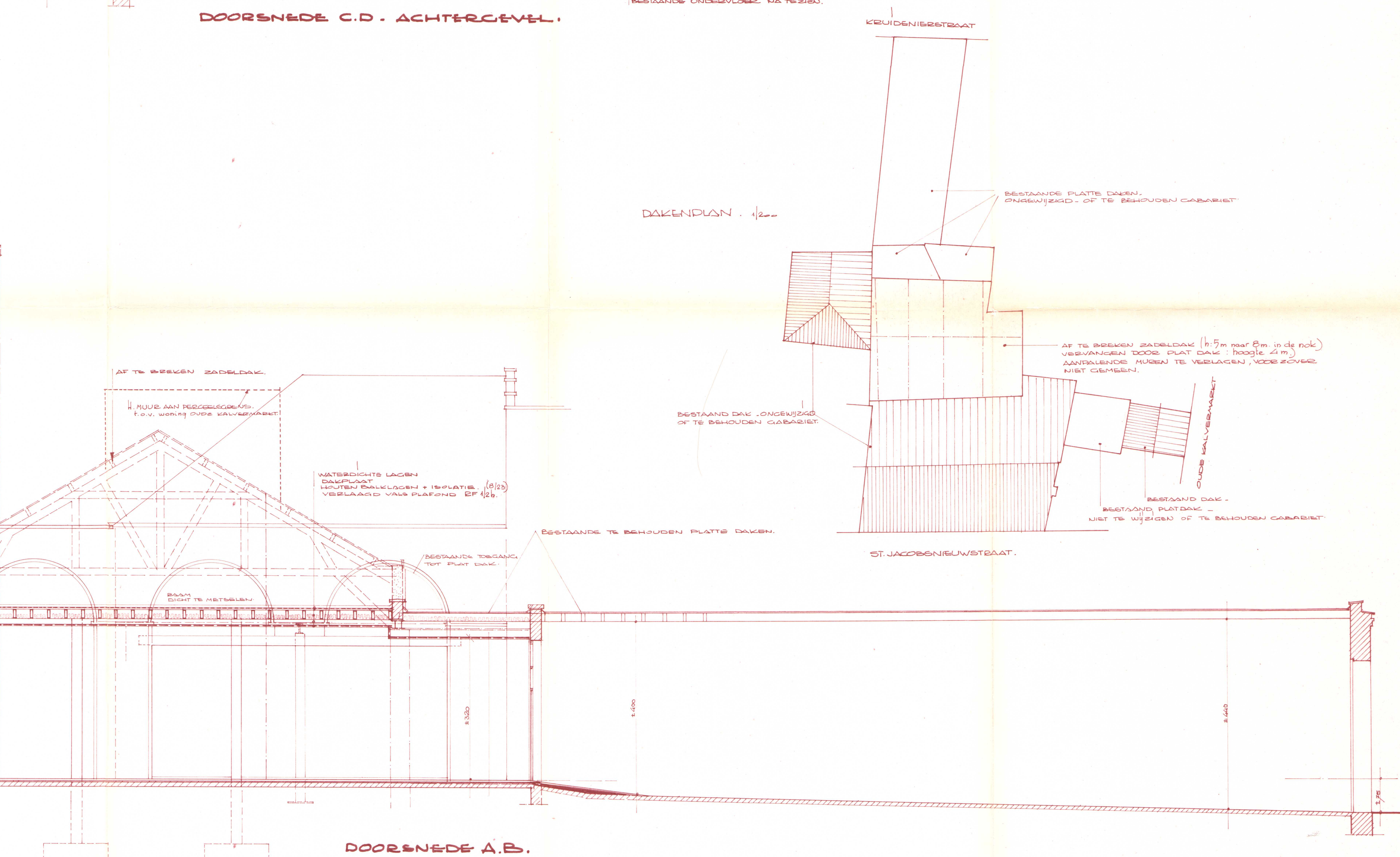
DOORSNEDEN B-B
