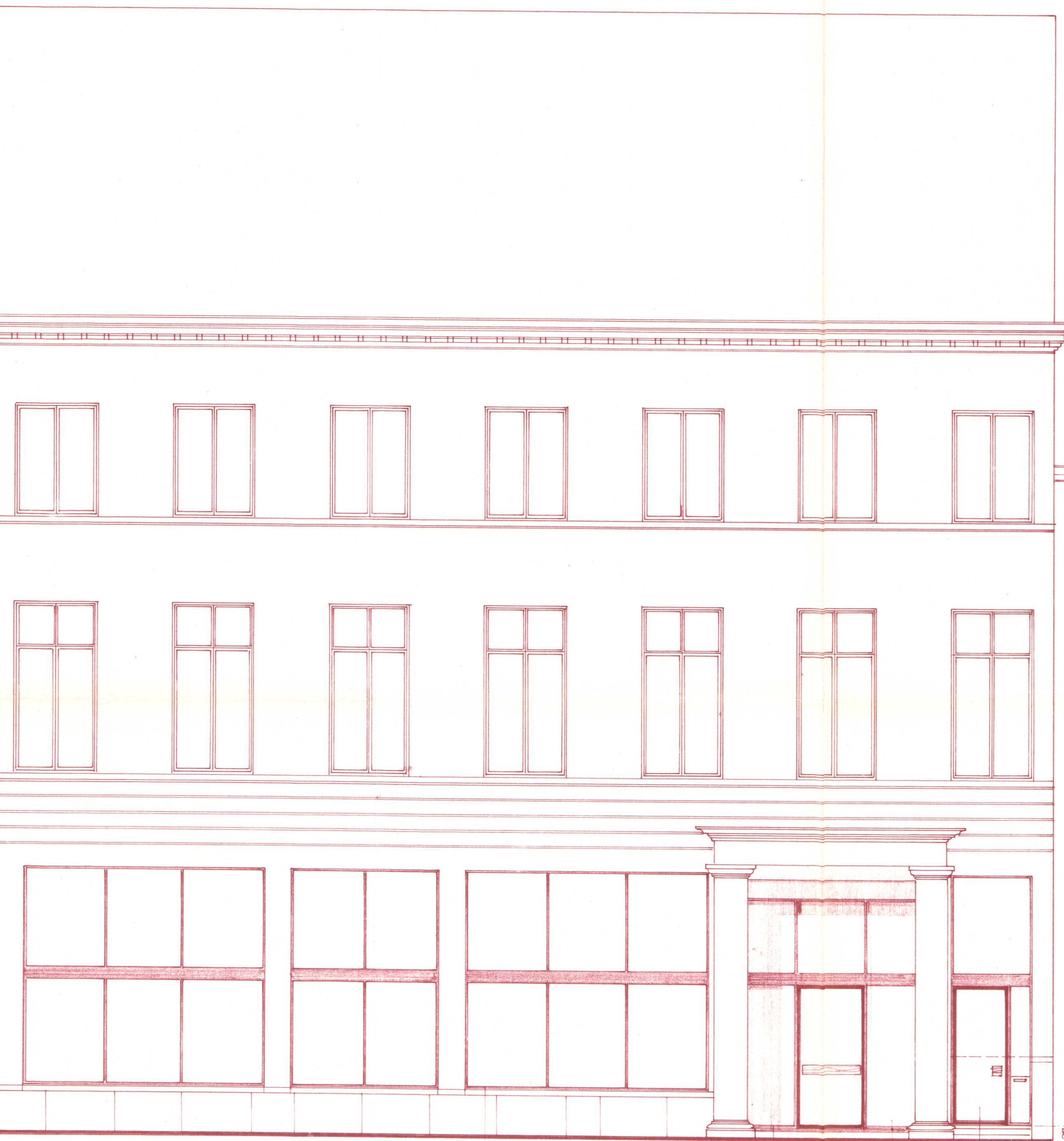
VOORGEVEL.
