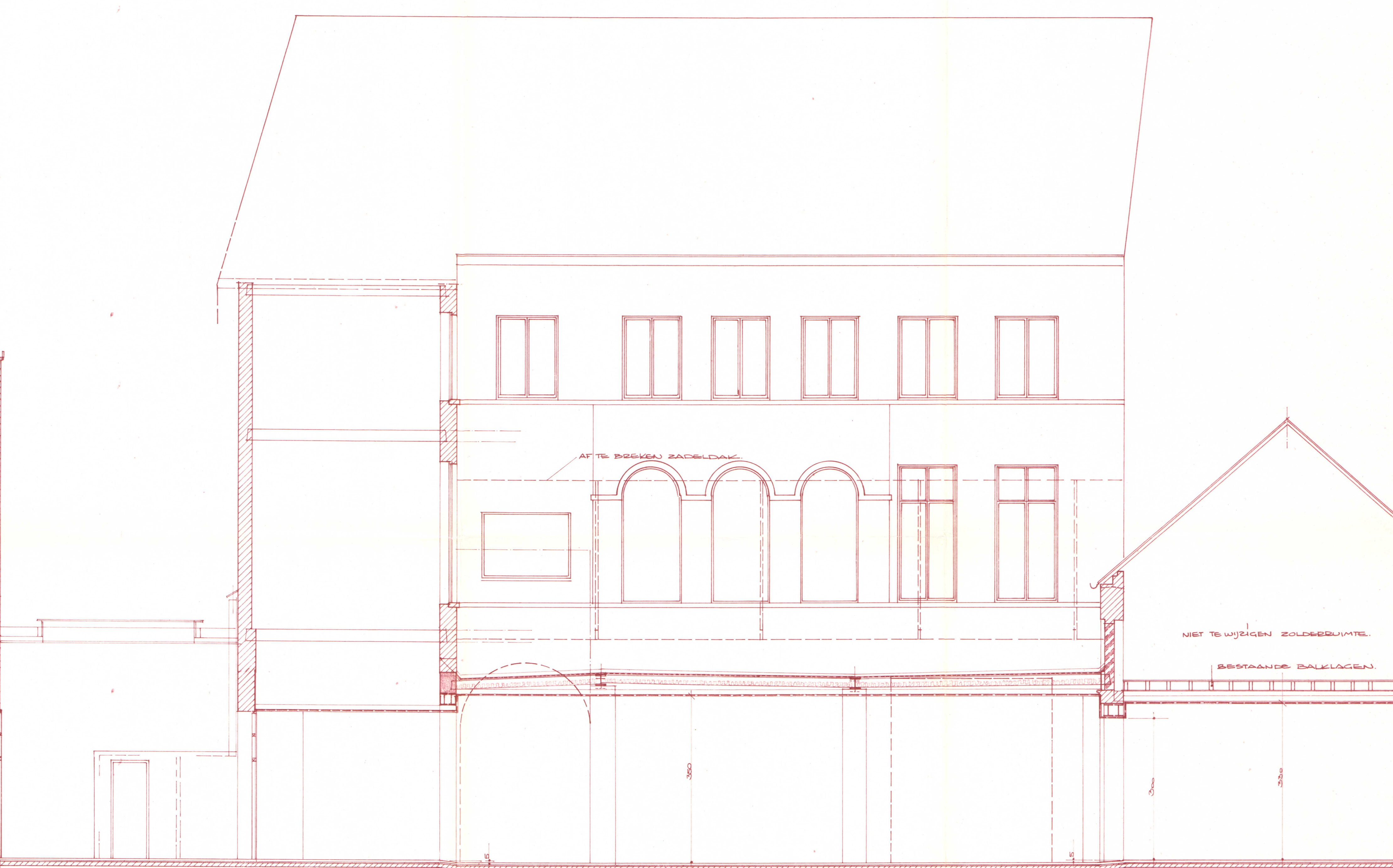
DOORSNEDEN C.D. - ACHTERGEVEL.
