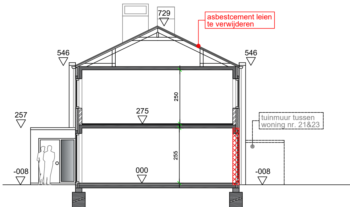
BESTAAND SNEDE AA
