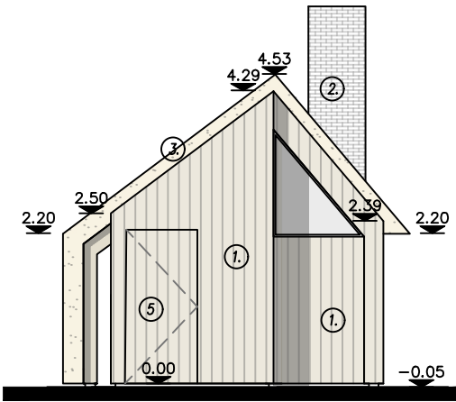
ZIJGEVEL RECHTS NIEUWE TOESTAND schaal 1/100
