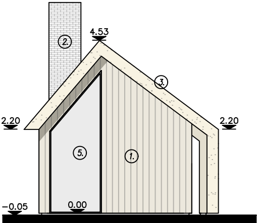
ZIJGEVEL LINKS NIEUWE TOESTAND schaal 1/100
