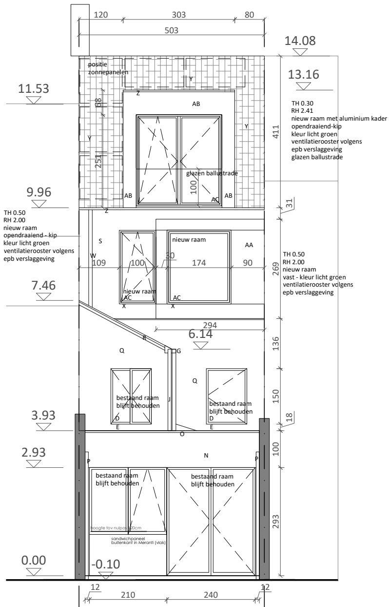
NIEUWE TOESTAND ACHTERGEVEL schaal 1-100
