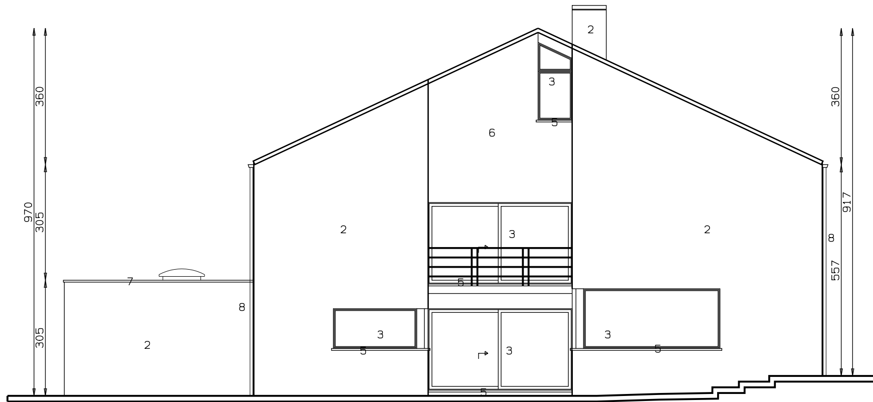
ZIJGEVEL RECHTS 1/100
