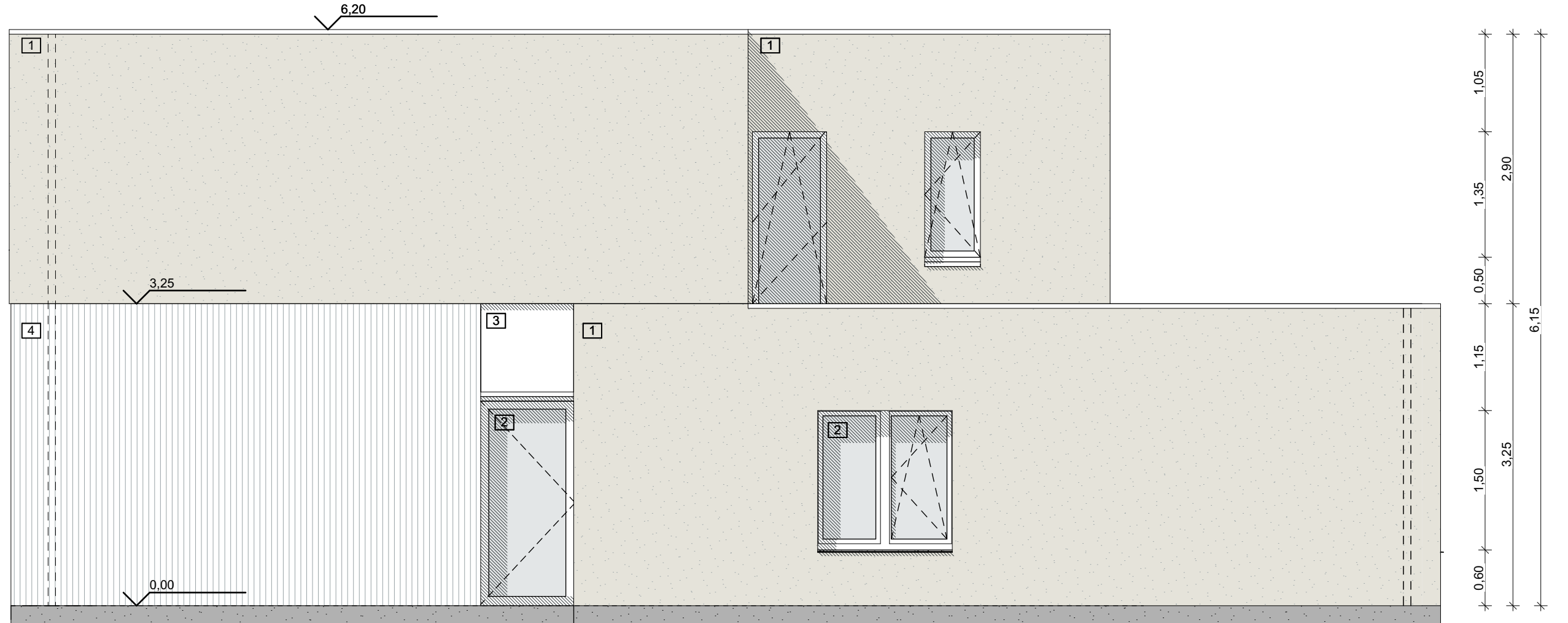
RECHTER ZIJGEVEL, nieuwe toestand schaal 1/50, maataanduiding in meter.
