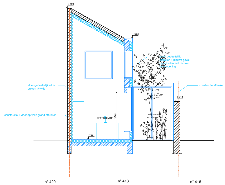
SNEDE FF nieuwe toestand schaal 1.100 eenheid: cm
