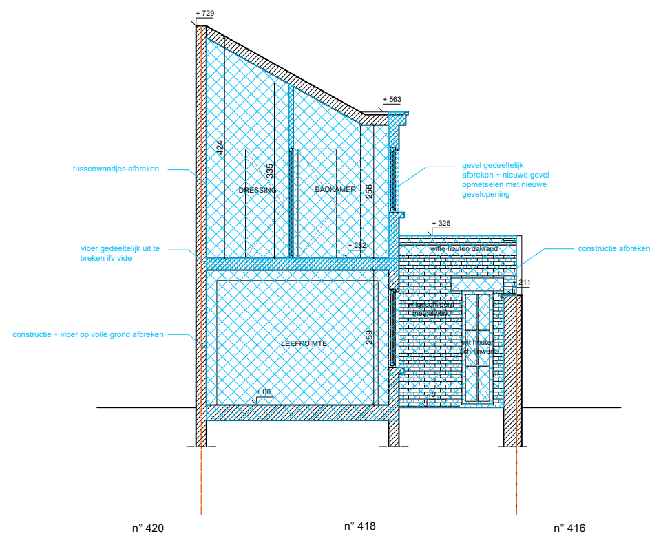
SNEDE FF bestaande toestand schaal 1.100 eenheid: cm
