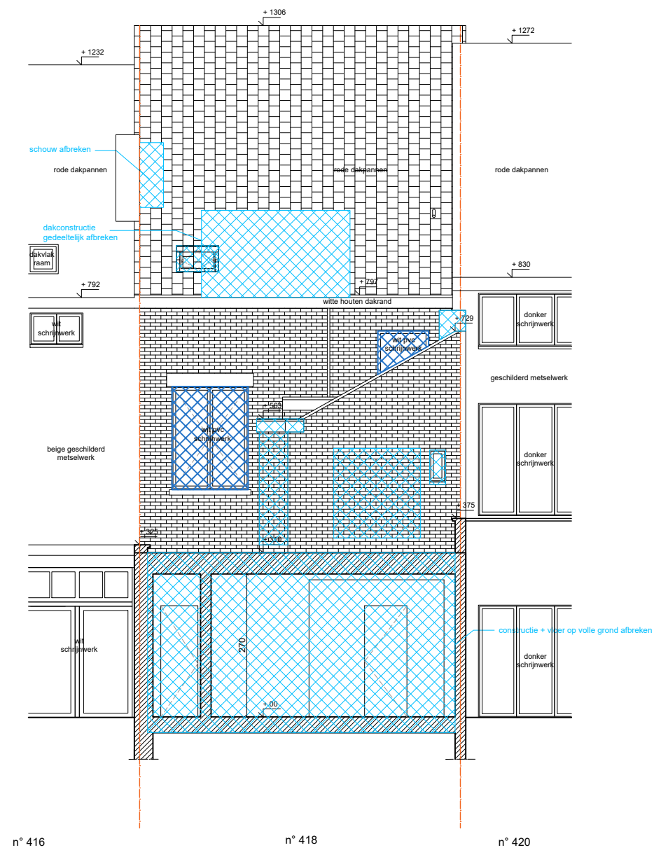
SNEDE EE bestaande toestand schaal 1.100 eenheid: cm
