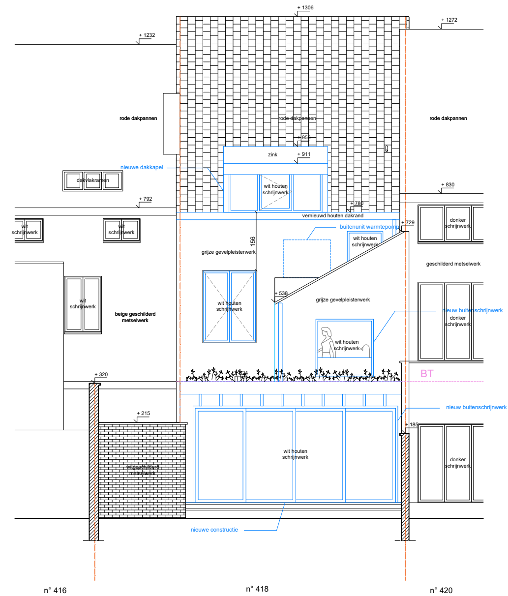
ACHTERGEVEL nieuwe toestand schaal 1.100 eenheid: cm
