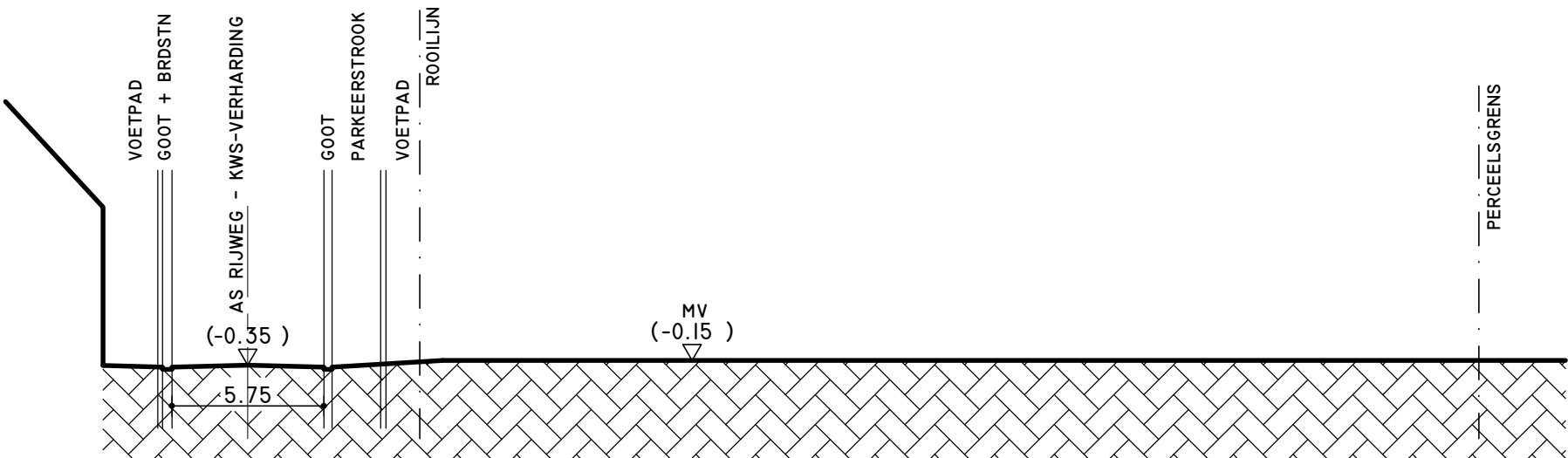
BESTAAND TERREINPROFIEL T-T
