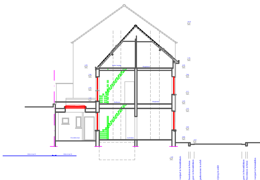
Terreinprofiel aa bestaande toestand schaal idem als inplantingsplan
