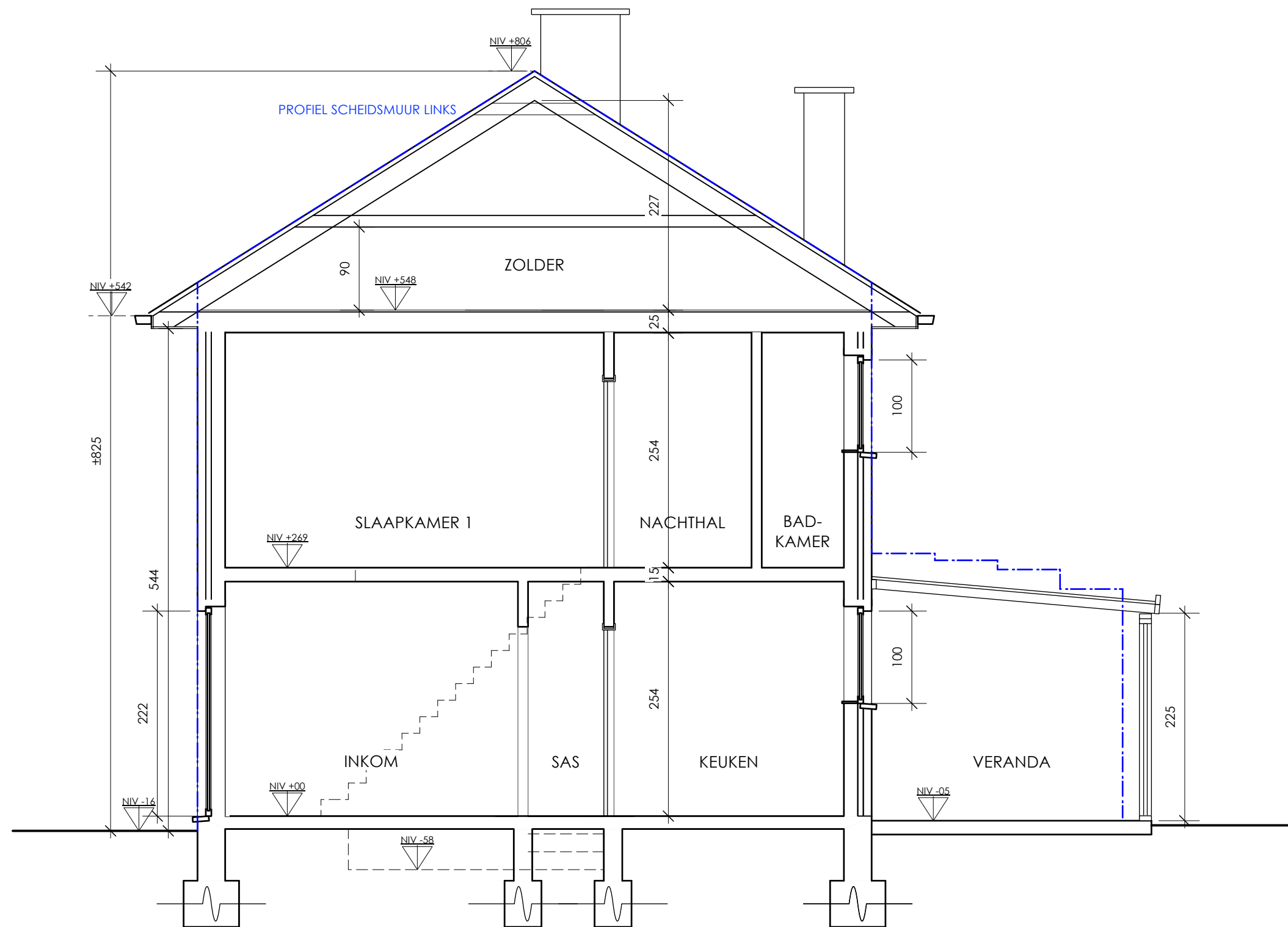
doorsnede AB (1:50)
