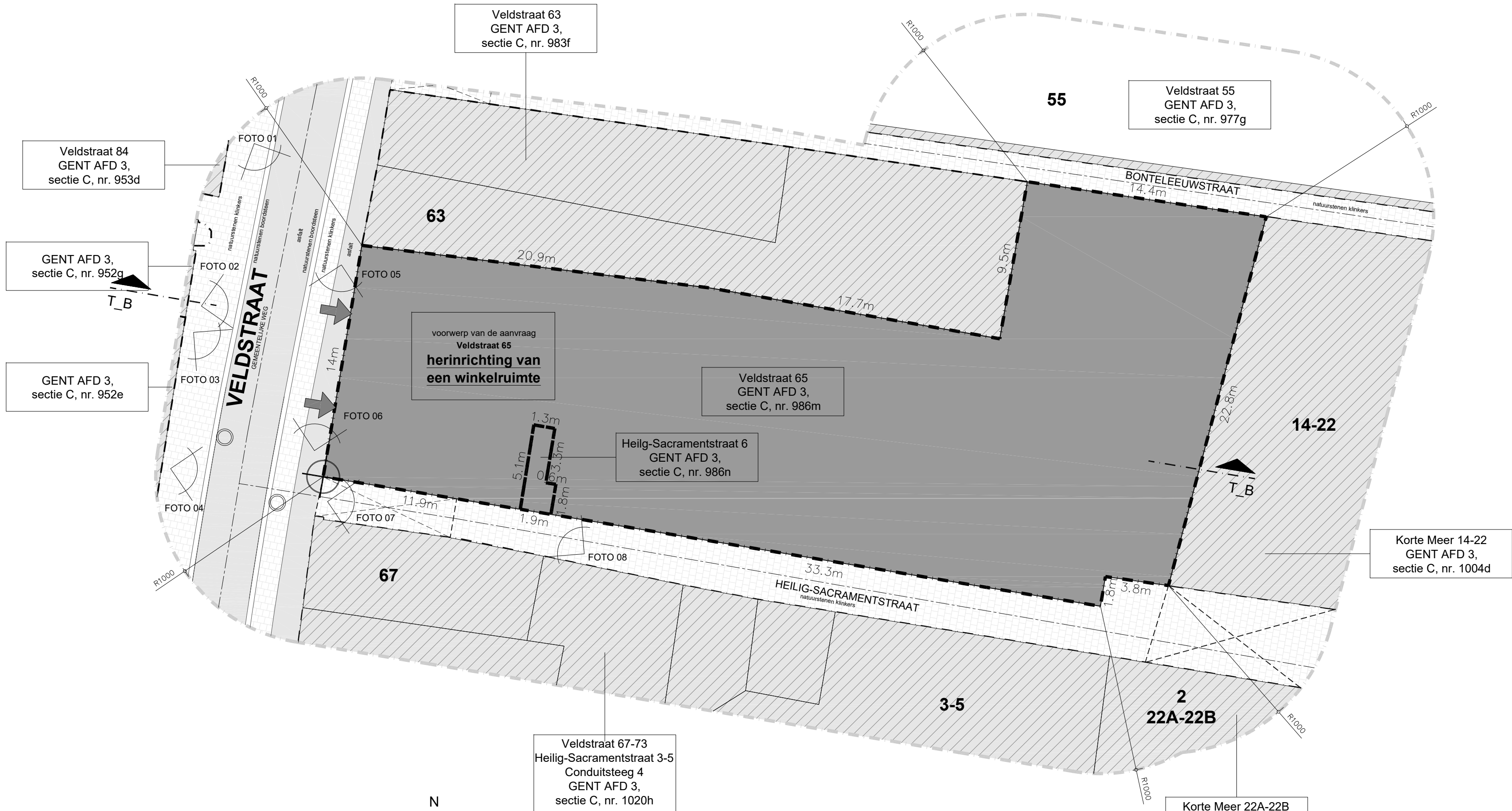
Inplantingsplan bestaande toestand SCHAAL 1 | 200
