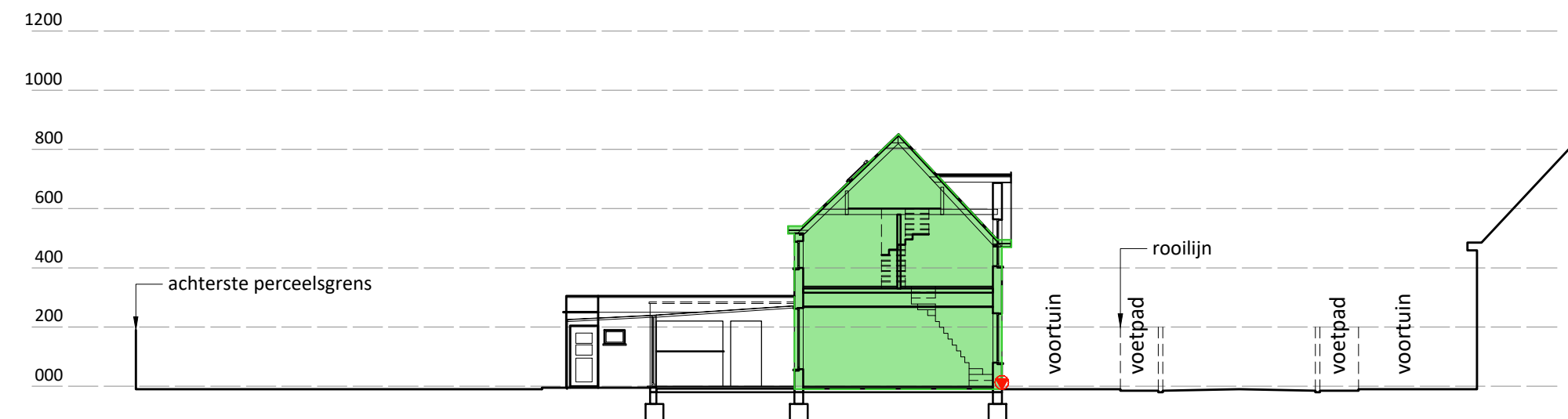
terreinprofiel 1 vergunde toestand schaal 1/200
