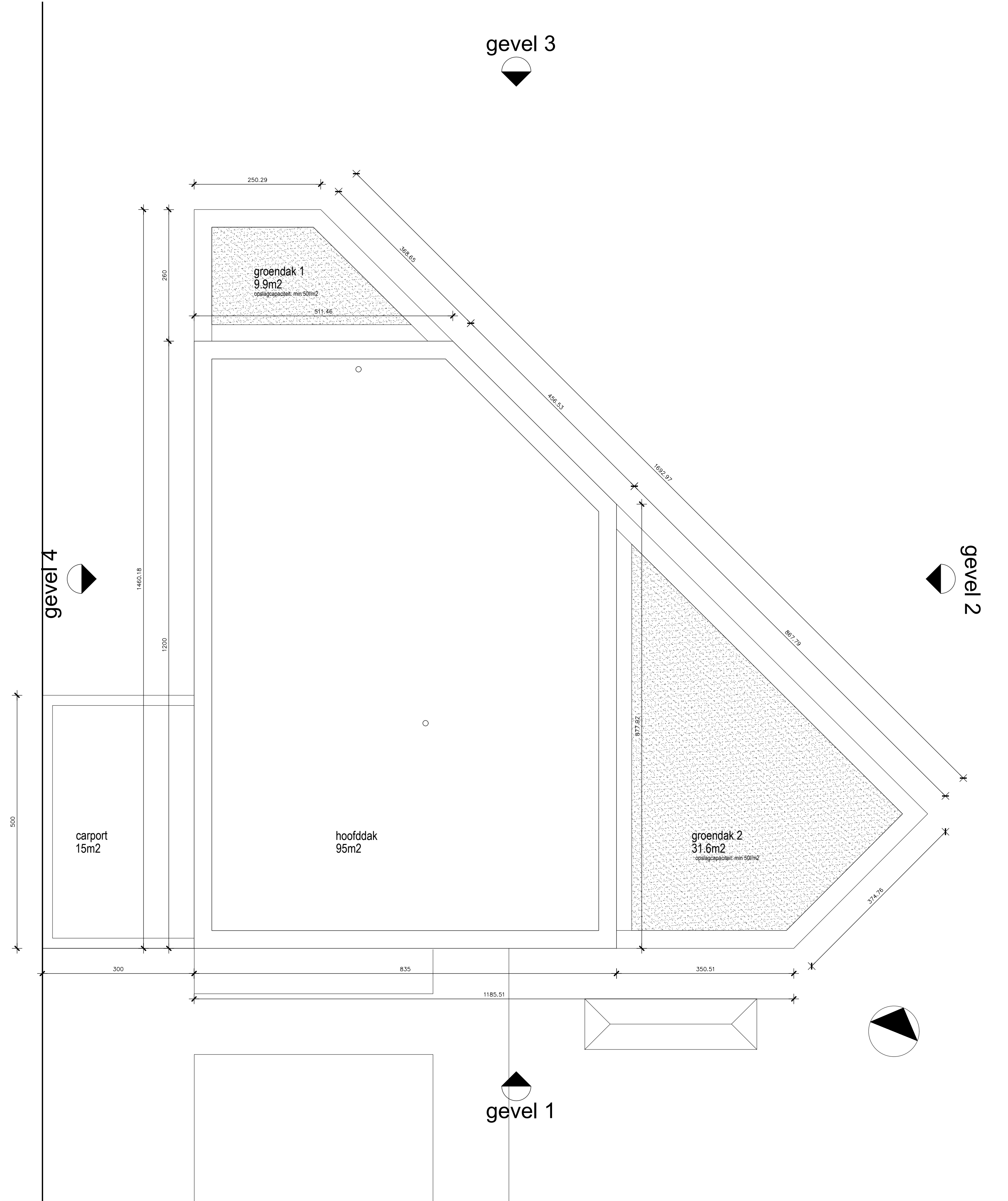
GRONDPLAN dakverdieping nieuwe toestand schaal: 1/50
