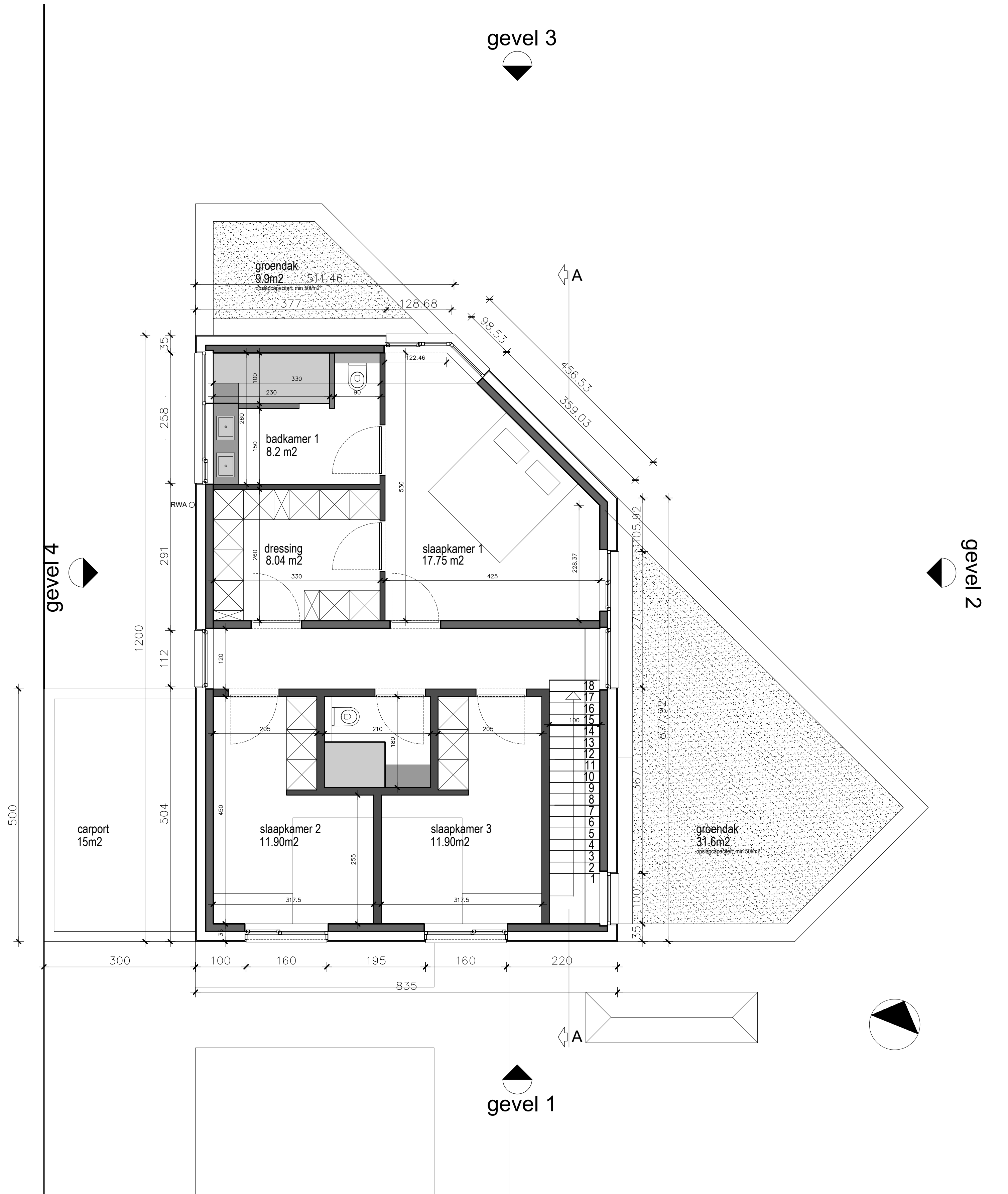
GRONDPLAN verdieping 1 nieuwe toestand schaal: 1/50
