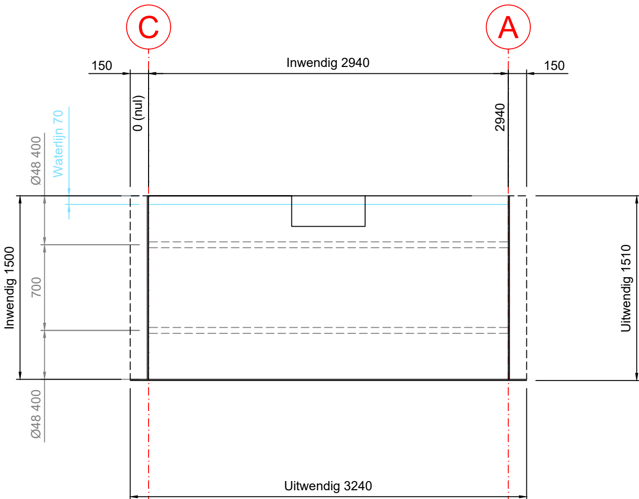
Binnenaanzicht D
