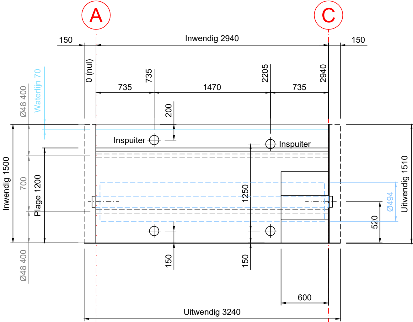
Binnenaanzicht B
