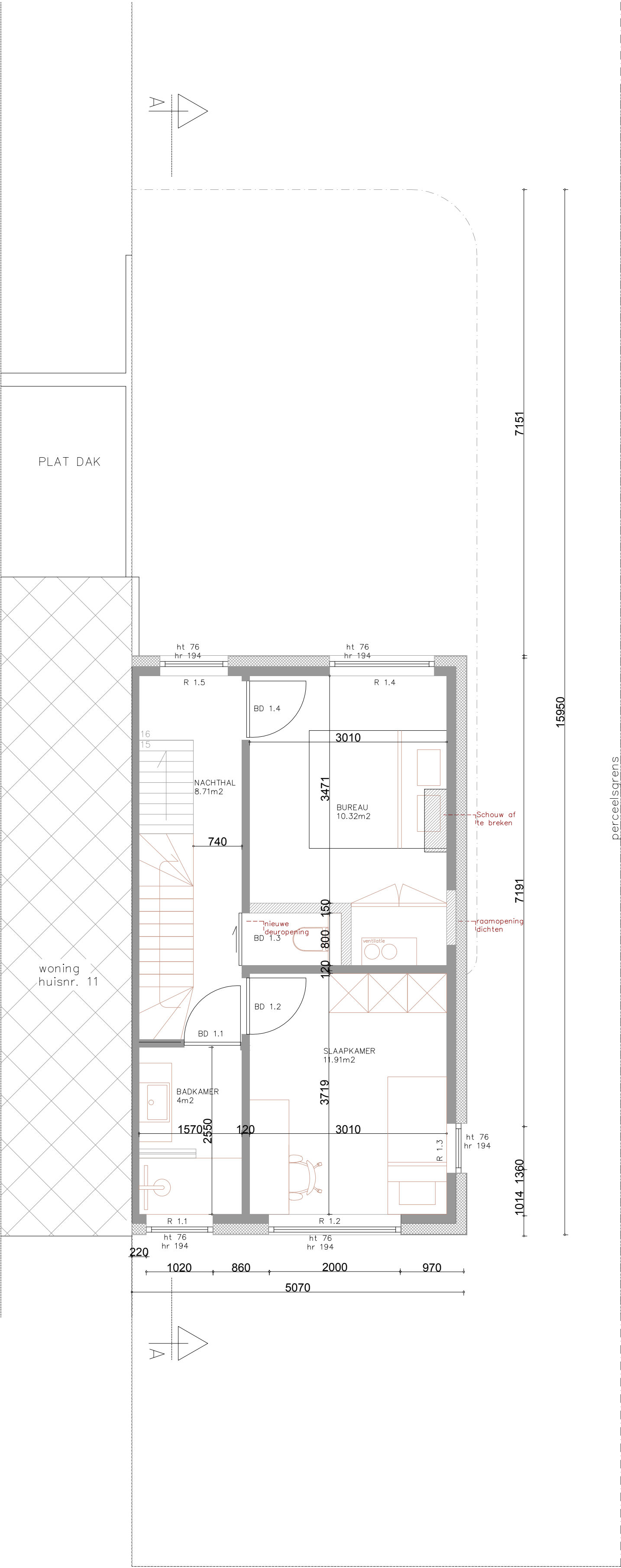
VERDIEPING +1 Nieuwe toestand schaal 1/50
