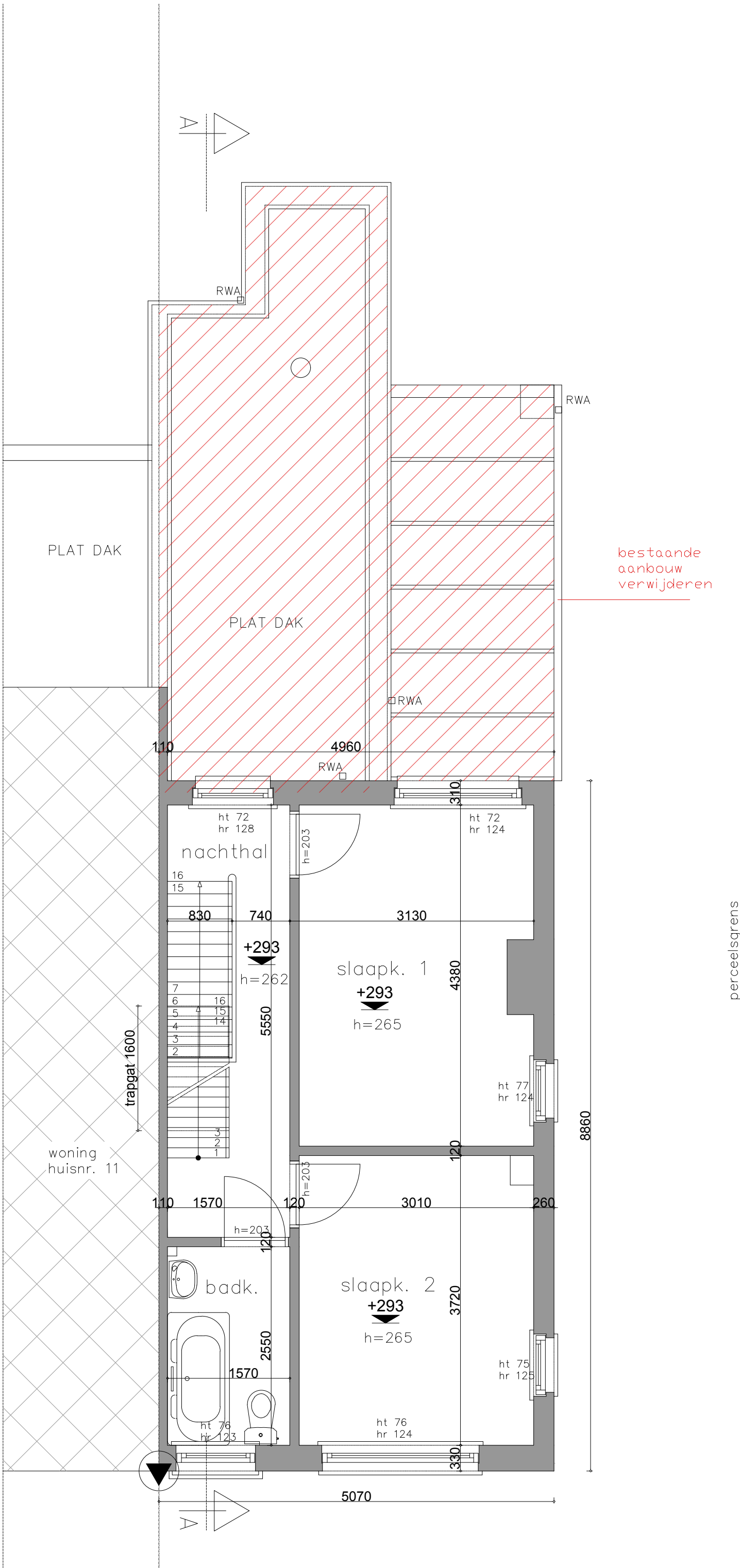
VERDIEPING +1 Bestaand toestand schaal 1/50
