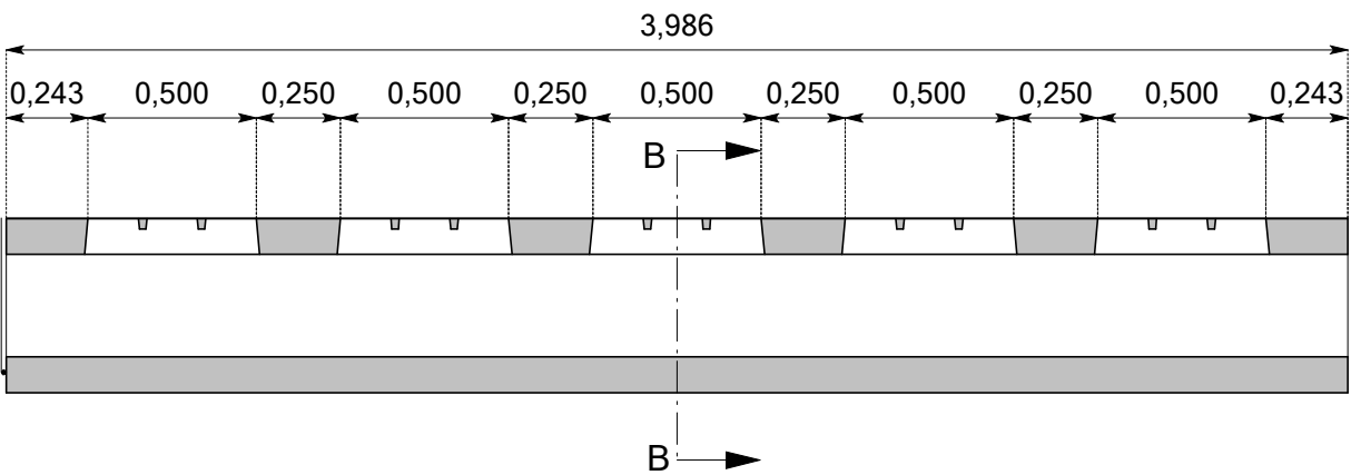
Bovenaanzicht
