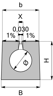
Doorsnede BB
