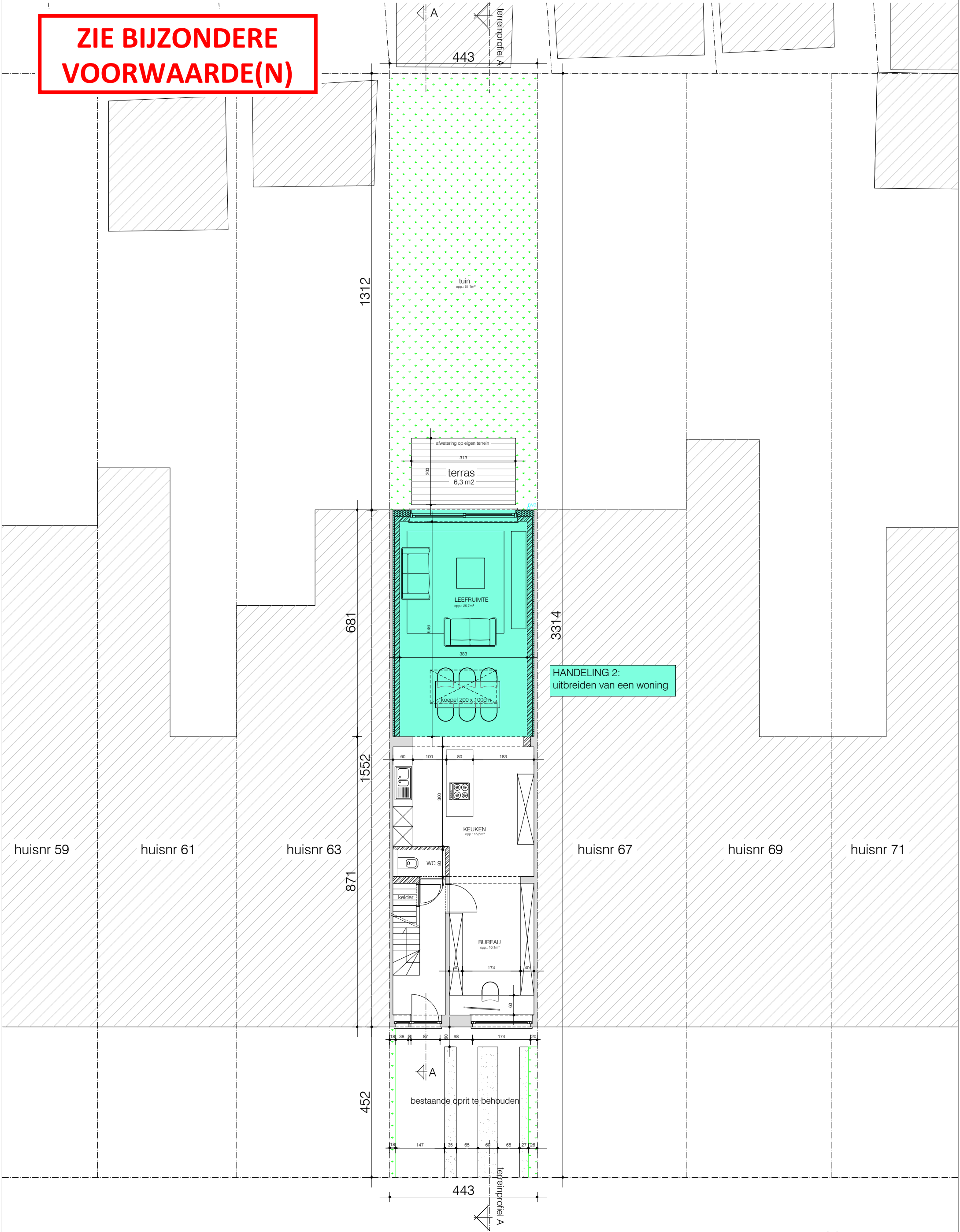
INPLANTINGSPLAN nieuwe toestand alle afmetingen zijn in cm
