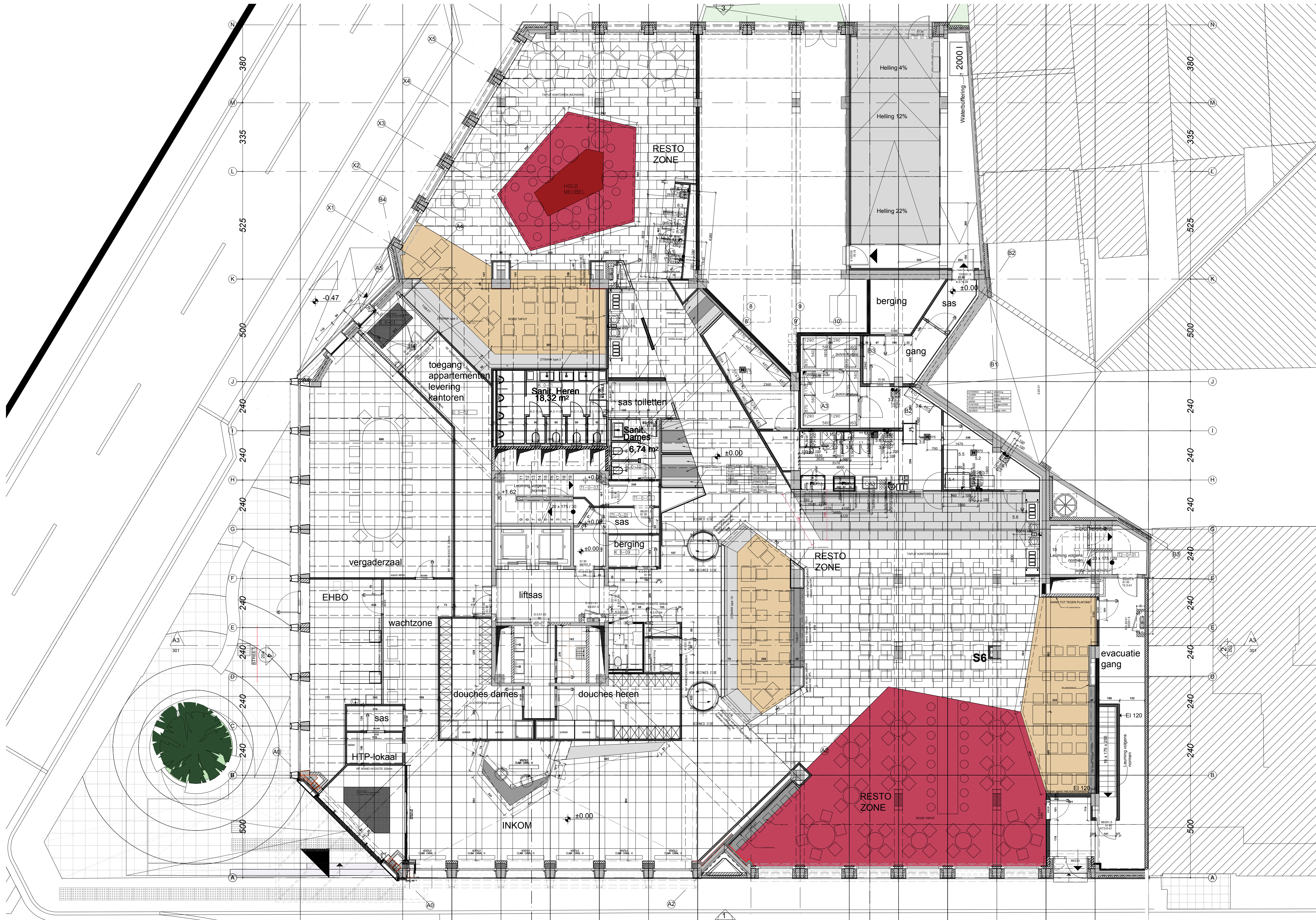
1 Grondplan bestaande situatie 05 Schaal: 1:100
