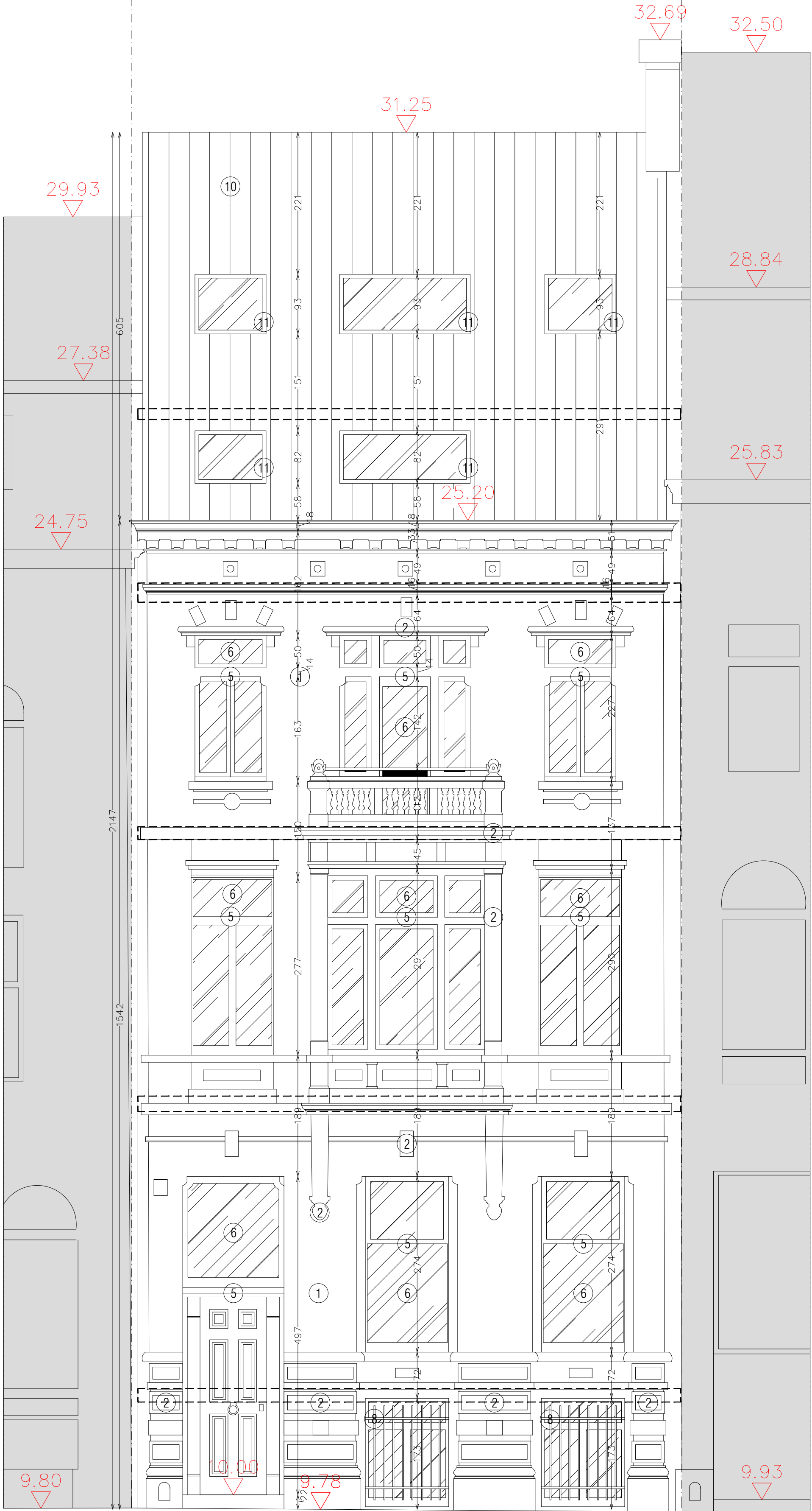
Kuiperskaai 6 Gevelaanzicht - voorgevel
