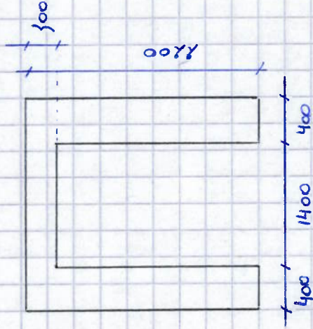
Voorraanzicht
