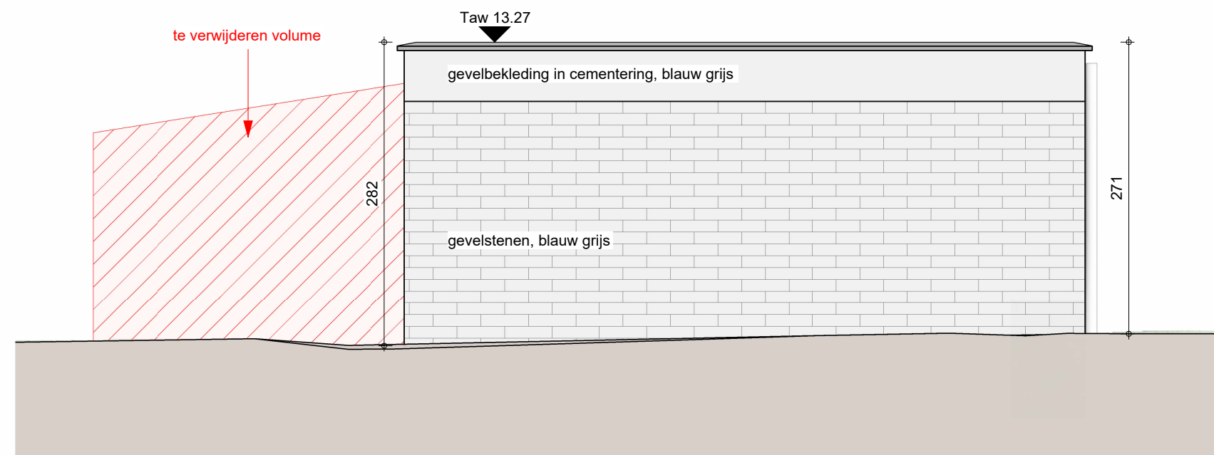
Tuinberging - Linkergevel BT
