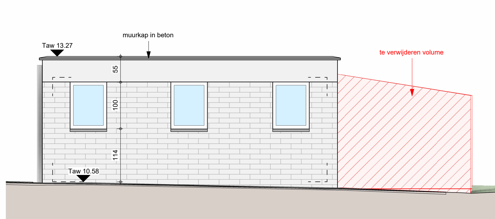
Tuinberging - Rechtergevel BT
