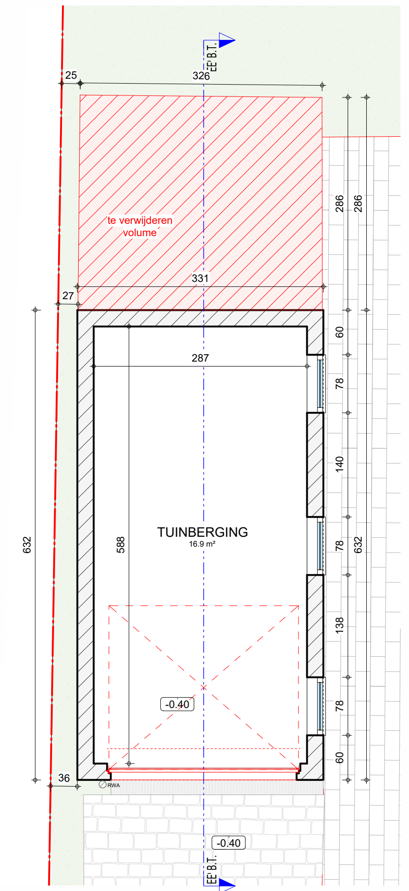
Grondplan Tuinberging BT
