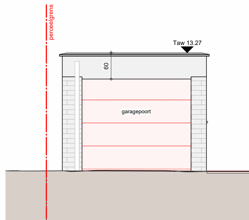
Tuinberging - Voorgevel BT
