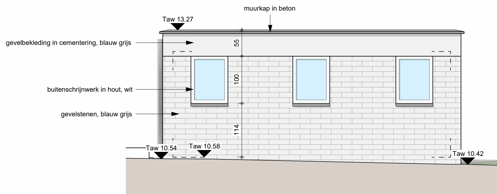
Tuinberging - Rechtergevel
