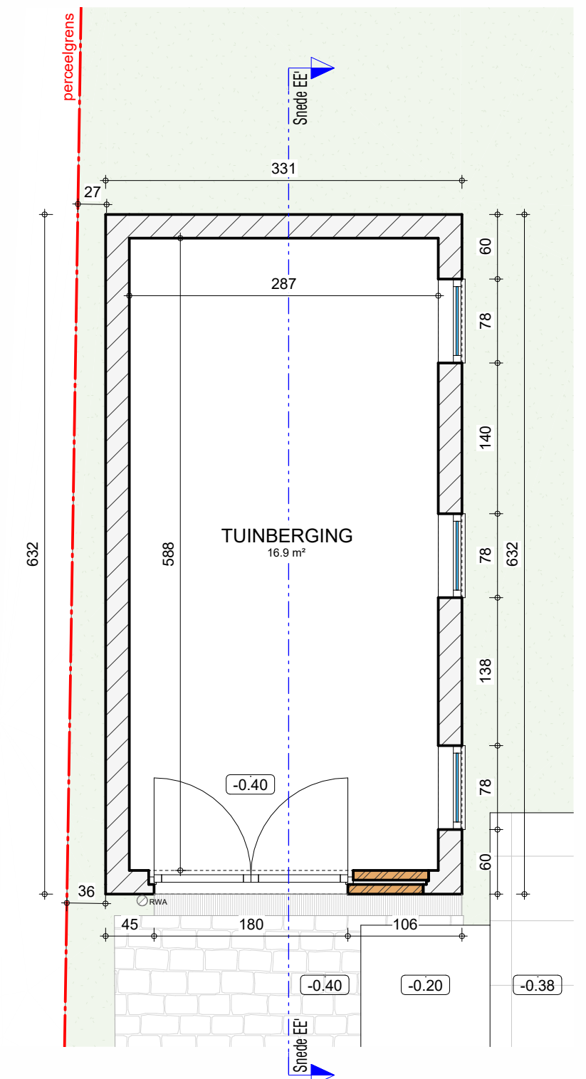
Grondplan Tuinberging
