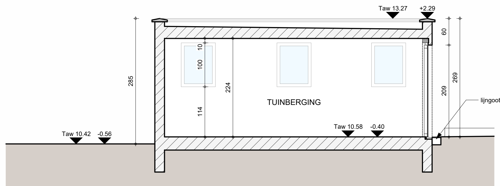
Snedede EE'
