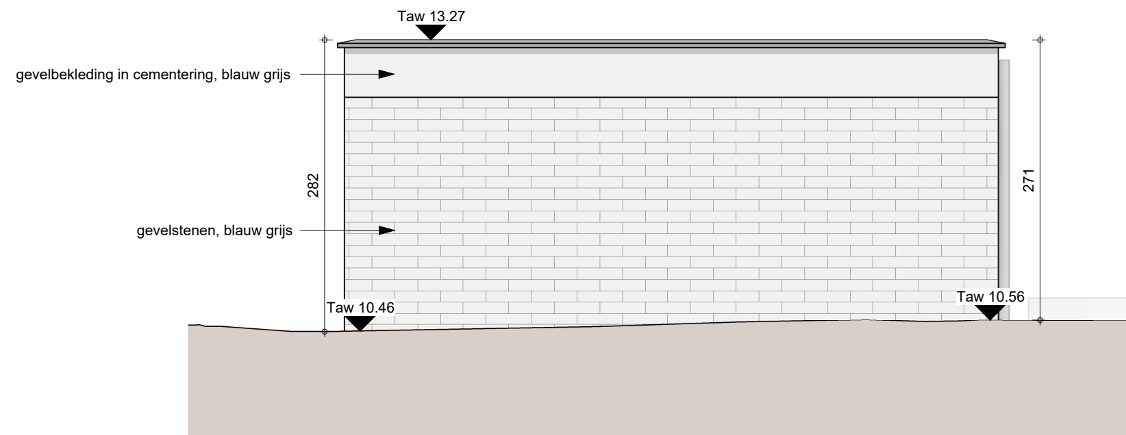
Tuinberging - Linkergevel
