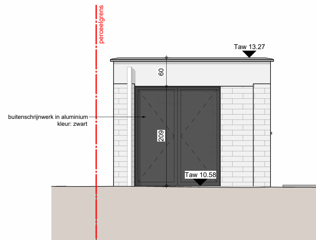
Tuinberging - Voorgevel
