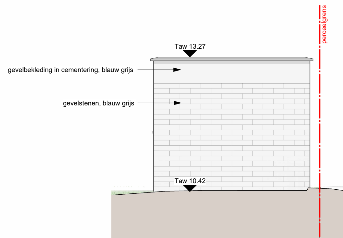
Tuinberging - Achtergevel
