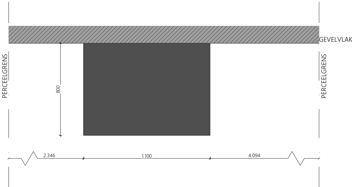
BOVENAANZICHT
