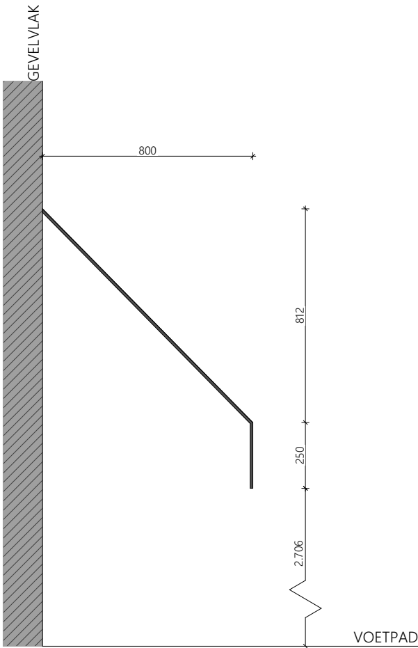
ZIJAANZICHT
