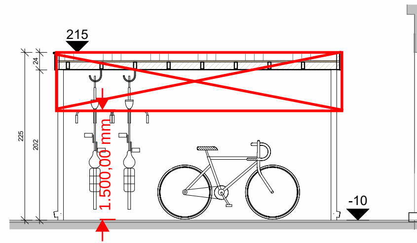
NT Doorsnede 4
