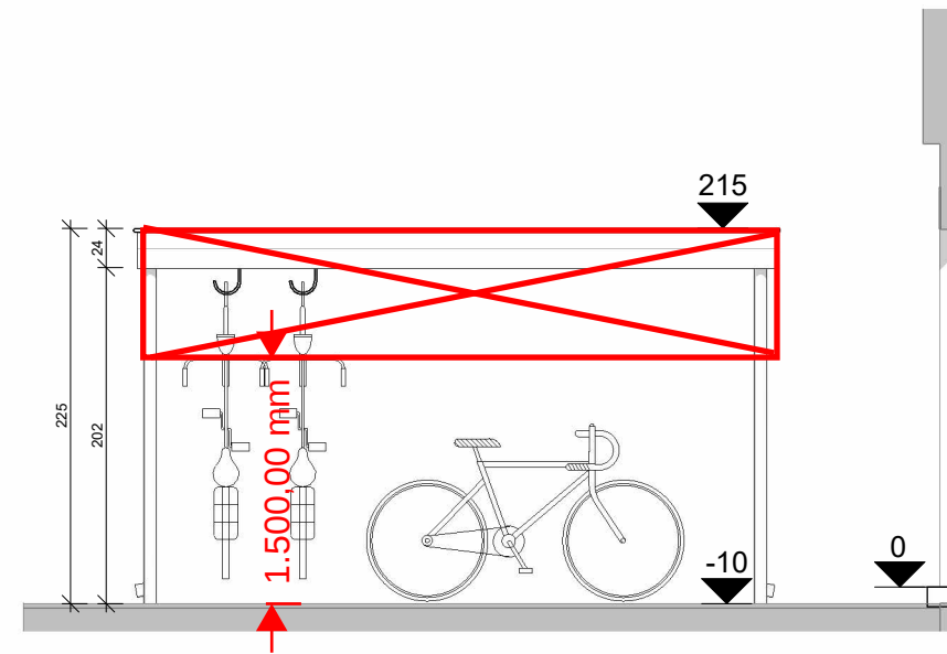
NT Zijgevel rechts fietsenstalling
