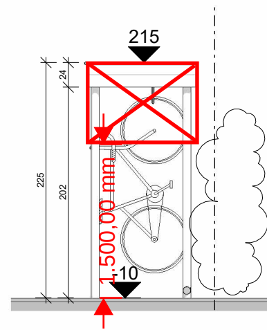
NT Achtergevel fietsenstalling
