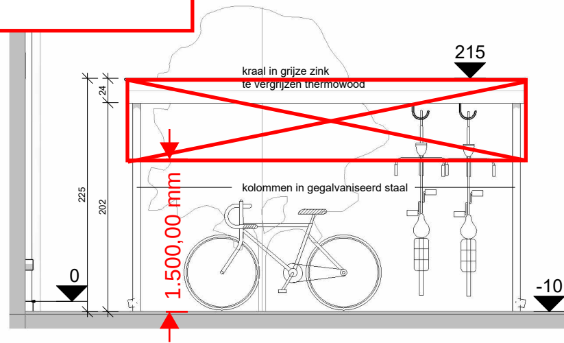
NT Zijgevel links fietsenstalling
