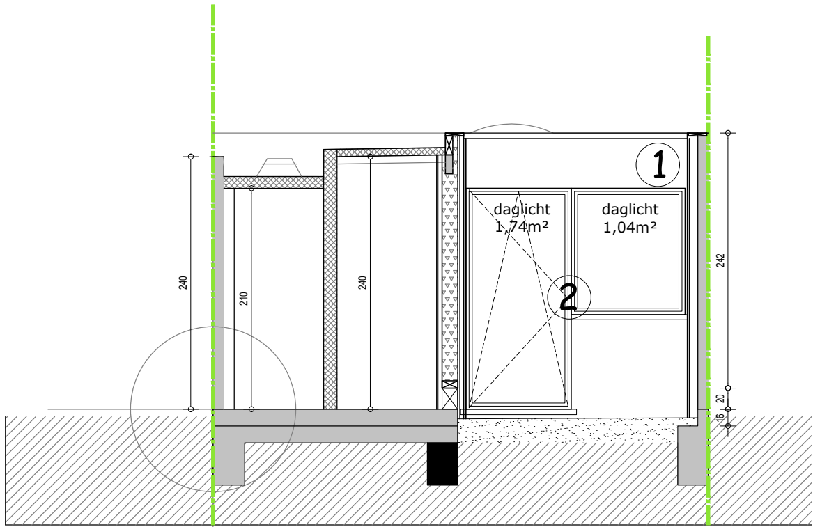
DOORSNEDE
