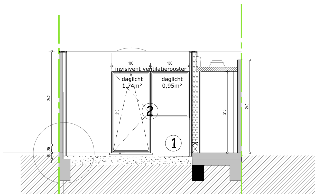
Gevel kamer 6
