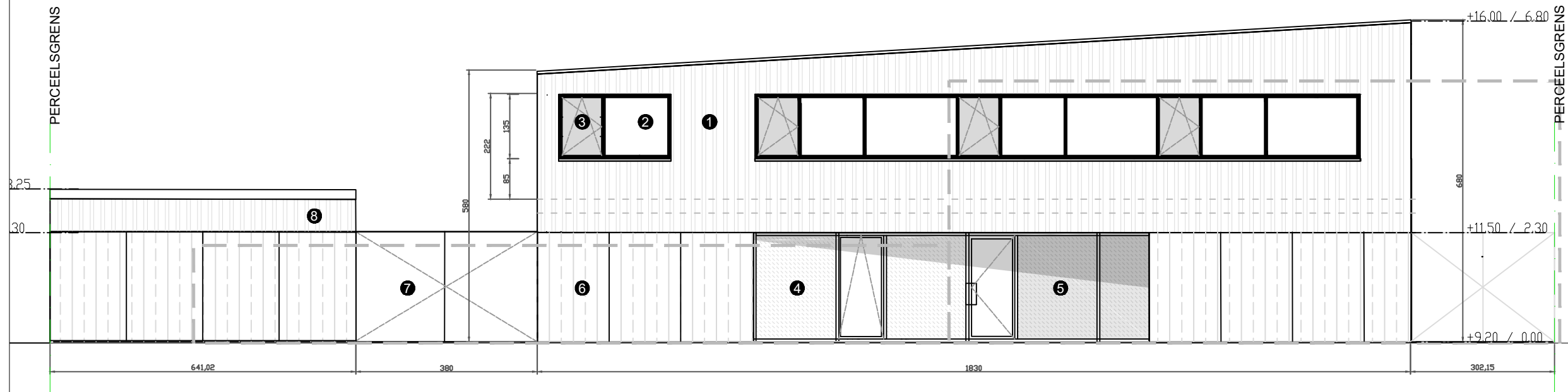
OOSTGEVEL - STRAATGEVEL
