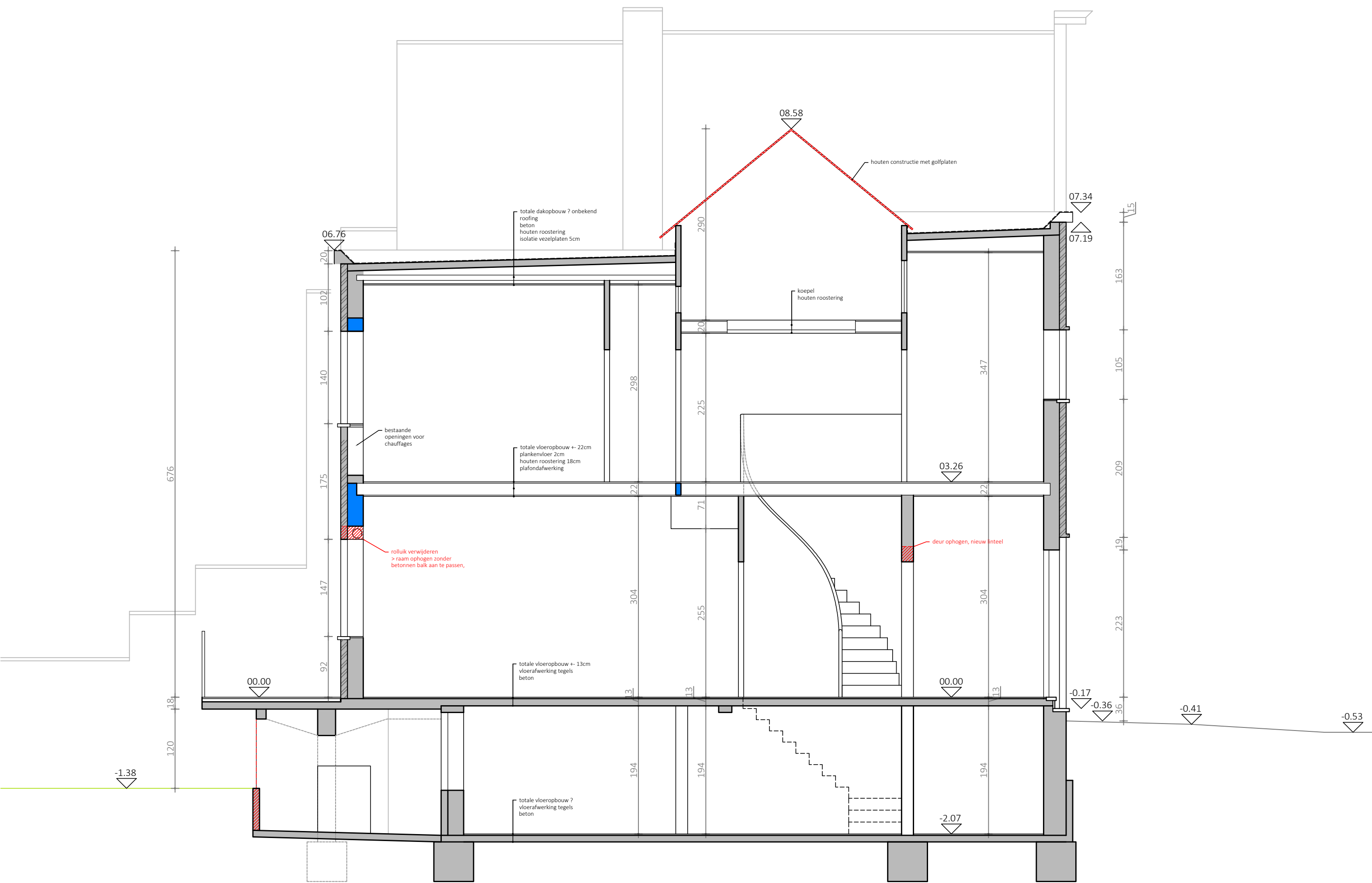
PRINCIPE SNEDE BB'
