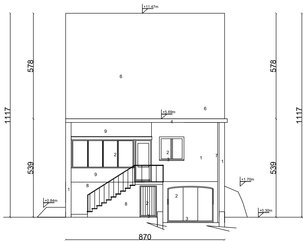
ACHTERGEVEL 1/100 Bestaande toestand
