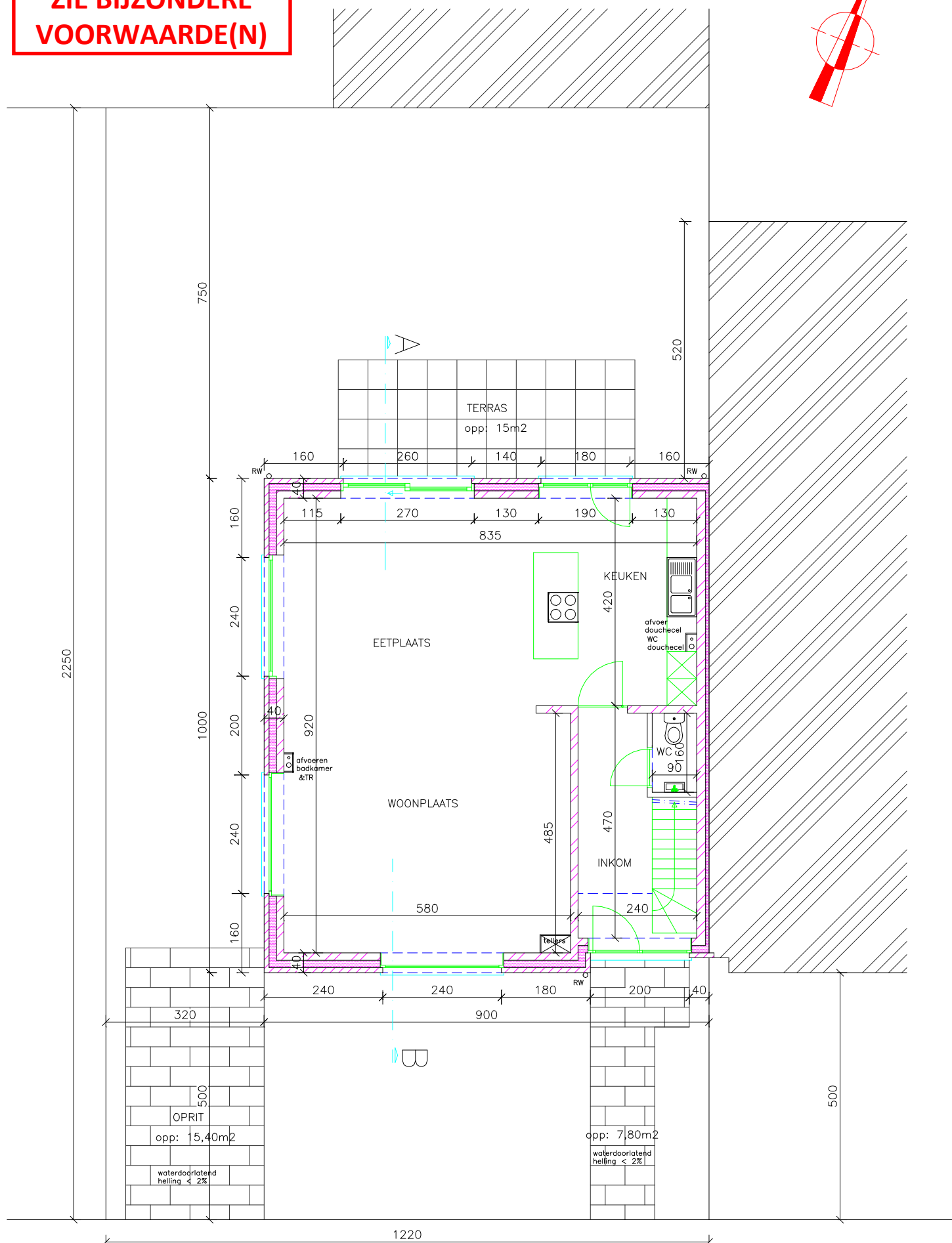
BA woning-P-N-1-gelijkvloers
