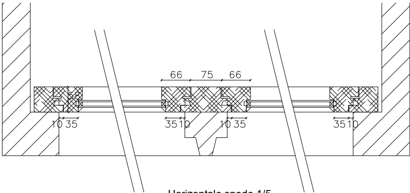
Horizontale snede 1/5
