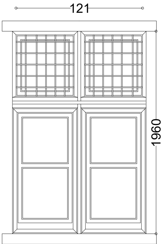
Vooraanzicht 1/20
