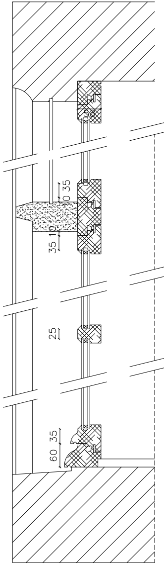
Verticale snede 1/5
