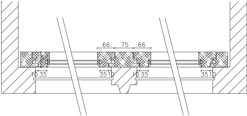
Horizontale snede (bovenlicht) 1/5
