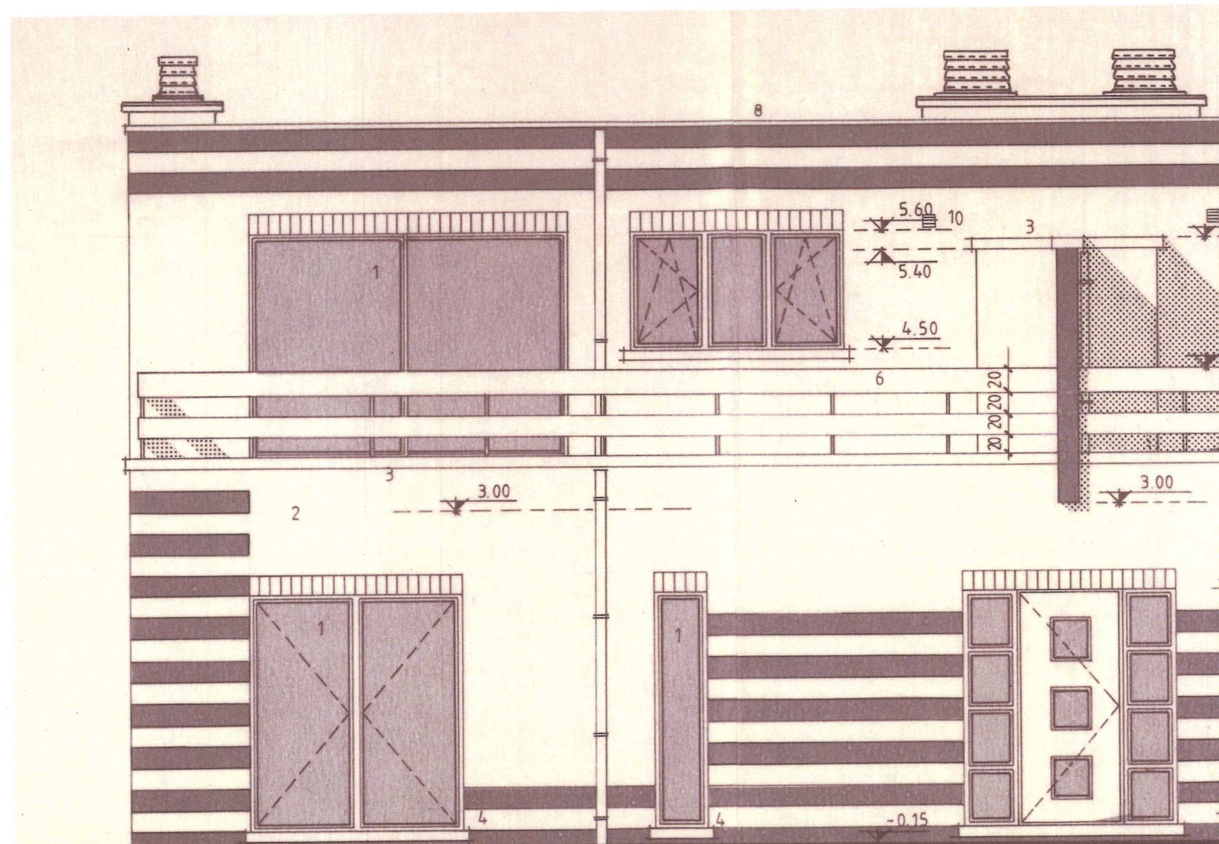
ACHTERAANZICHT BT schaal 1/50
