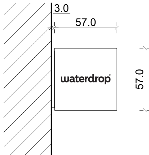
Zij-aanzicht
